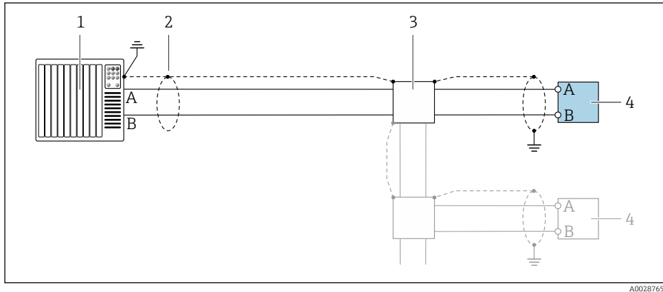
16 Anschlussbeispiel für Modbus RS485, nicht explosionsgefährdeter Bereich und Zone 2/Div. 2
