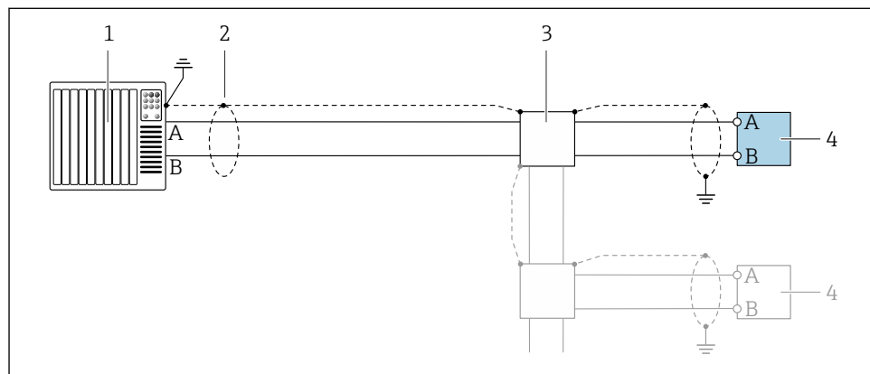
16 Příklad připojení pro PROFIBUS DP, prostředí bez nebezpečí výbuchu a zóna 2 / div. 2
