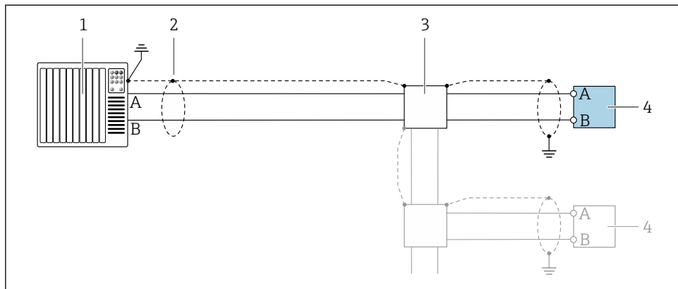
16 Aansluitvoorbeeld voor PROFIBUS DP explosieveilige omgeving en zone 2/Div. 2
