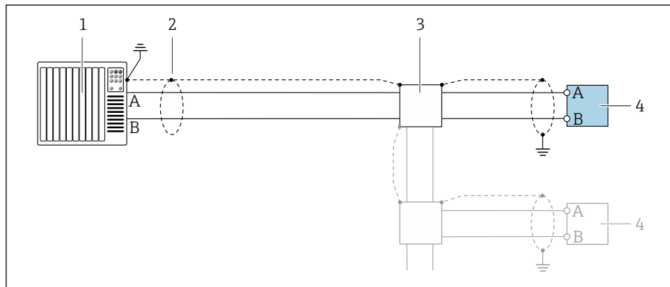
16 Exemplu de conexiune pentru PROFIBUS DP, zonă care nu prezintă pericol și zona 2/div. 2
