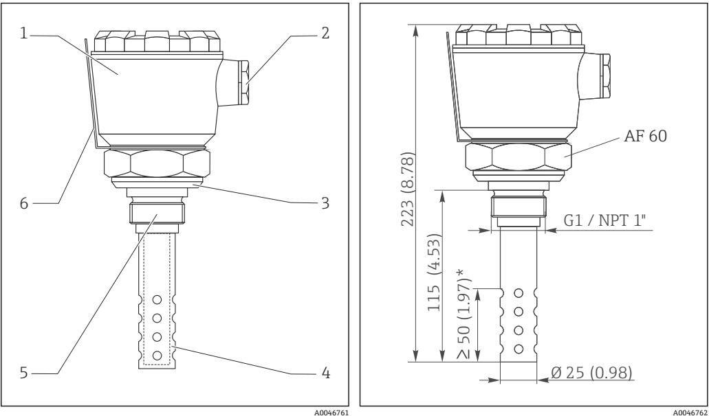
図 5 構造
