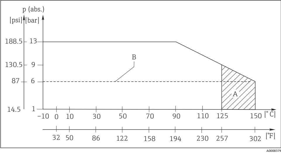
图 9 温度-压力曲线
