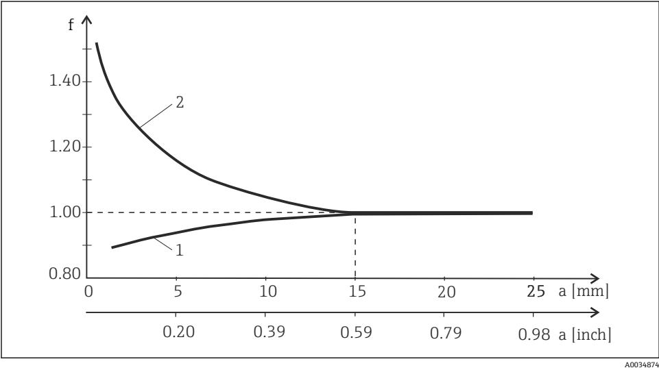
图 6 安装系数 (f) 和传感器与管壁间距离 (a) 的关系示意图 1 导电性管壁 2 电绝缘管壁
