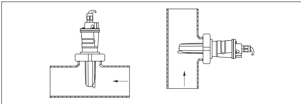
图 7 CLS54 的安装示意图，箭头指向与流向一致
