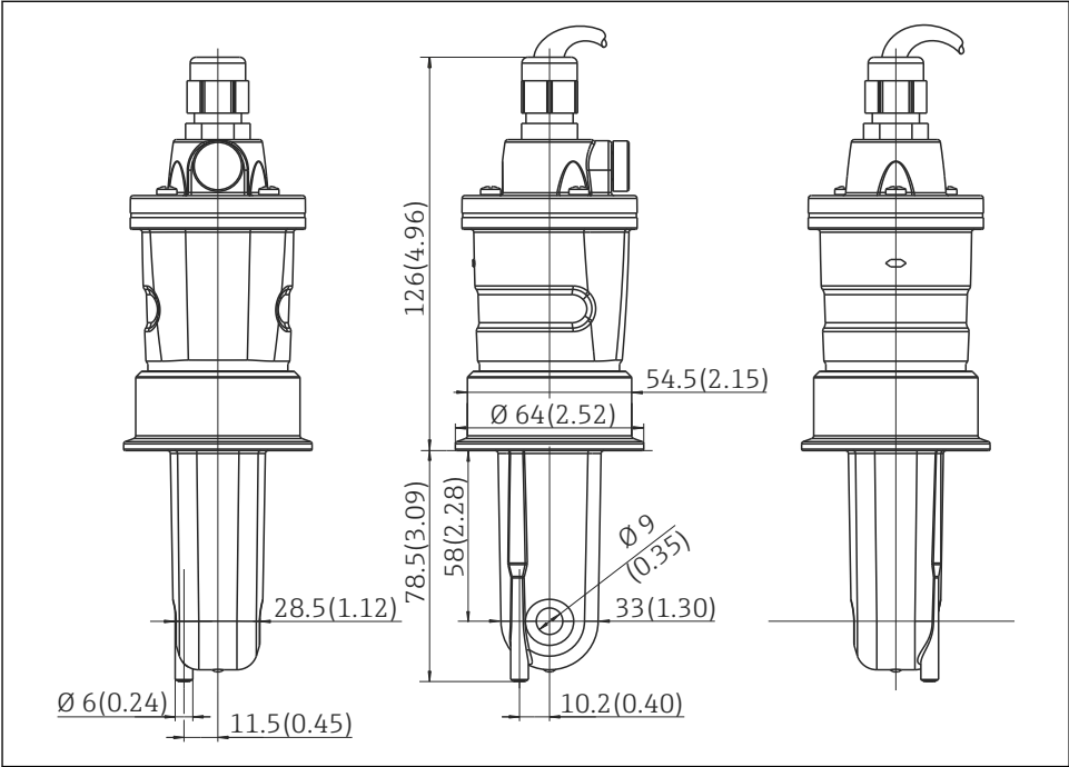
1 外形尺寸示意图(长型); 单位: mm (inch)
