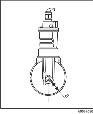
图 5 CLS54 的安装示意图 a 与管壁间的距离
