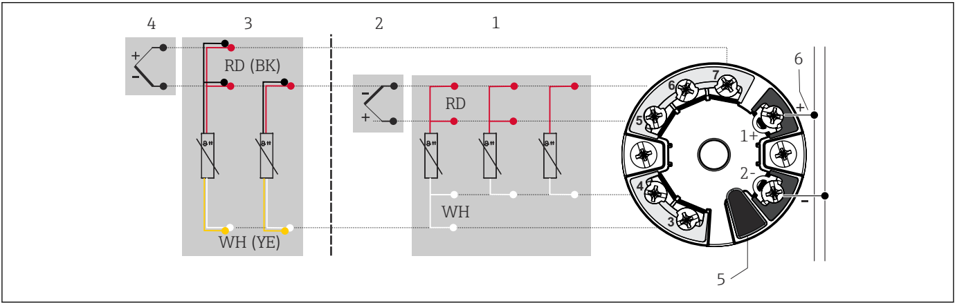
3 Klemmenanschlussbelegung des Kopftransmitters
