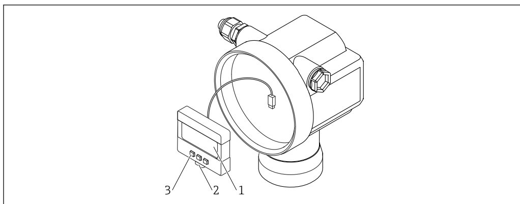
21 LCD-Modul im Gehäuse
