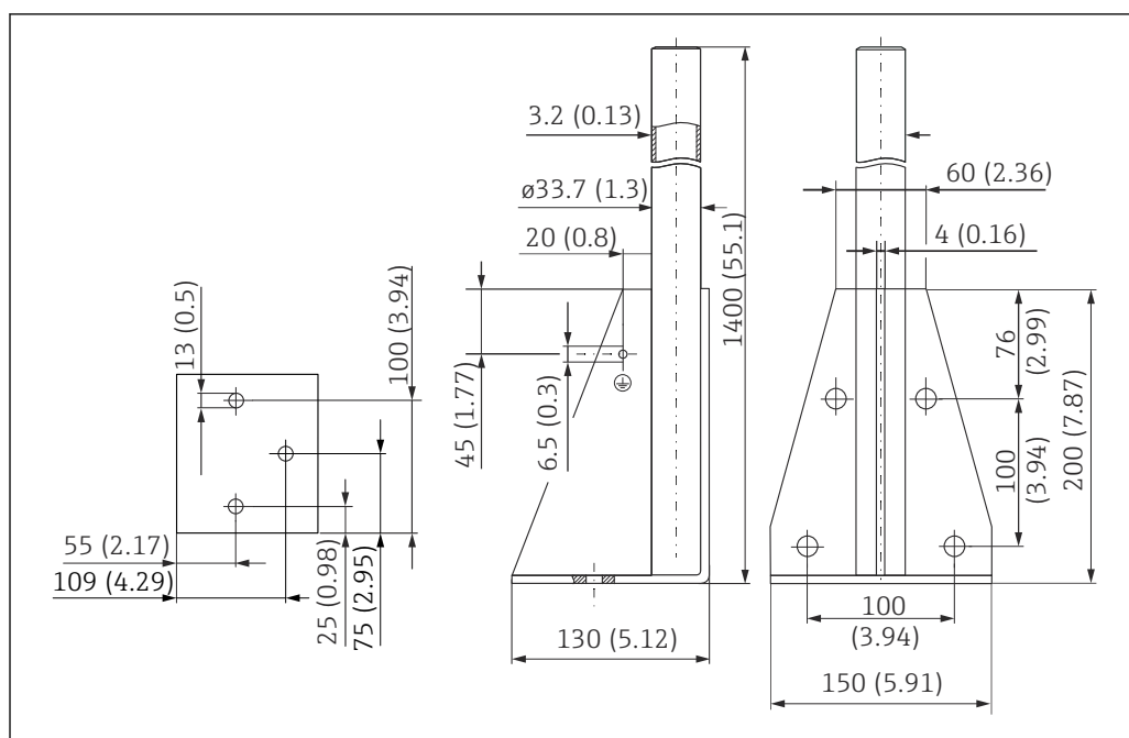
30 Abmessungen. Maßeinheit mm (in)
