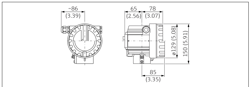
17 Abmessungen Gehäuse F12. Maßeinheit mm (in)
