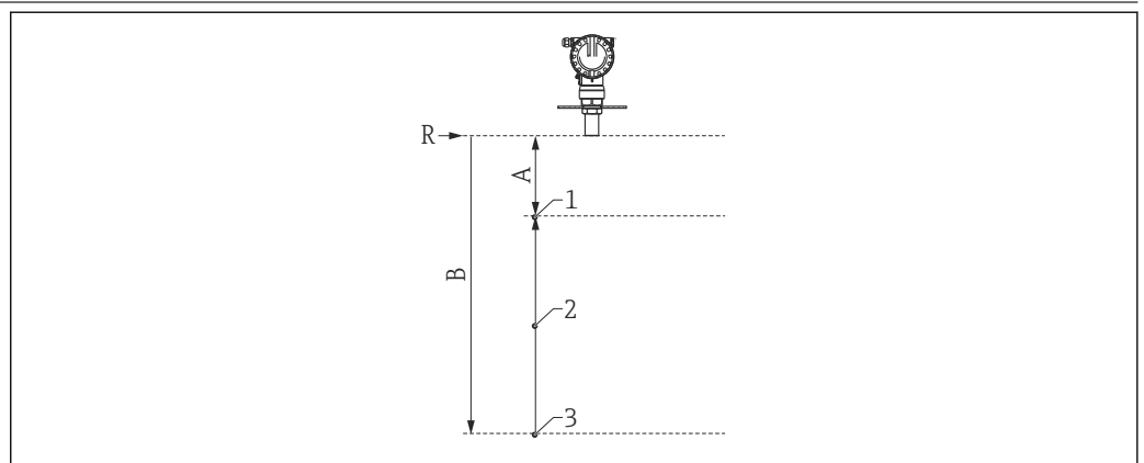
25 Beispiel Darstellung 3-Punkt-Linearitätsprotokoll
