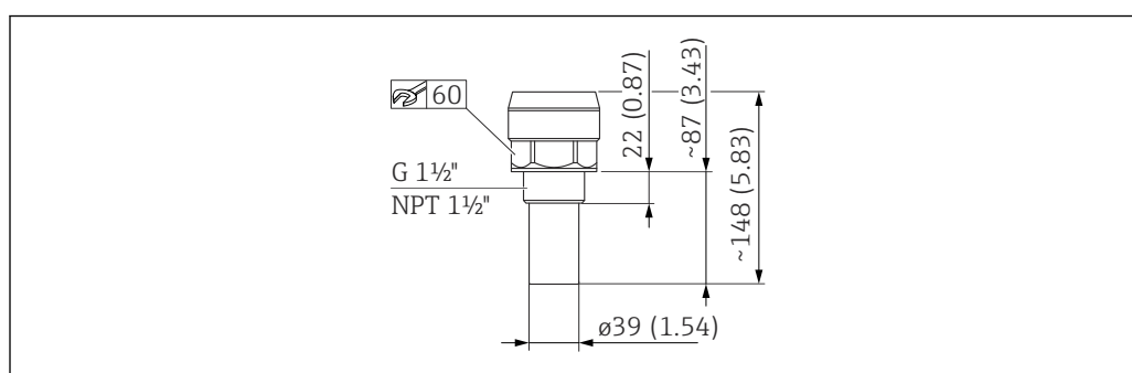
19 Abmessungen Sensor FMU40. Maßeinheit mm (in)
