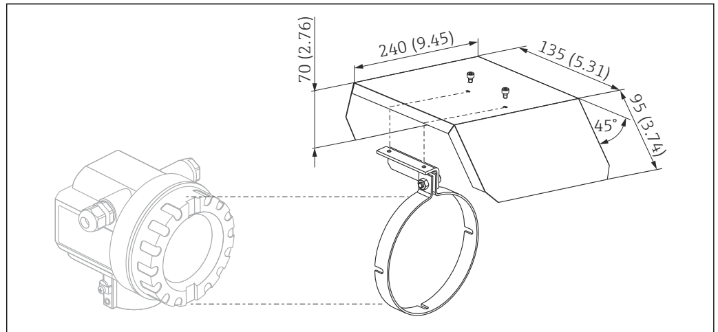
36 Wetterschutzhaube für Gehäuse F12 oder T12 . Maßeinheit mm (in)
