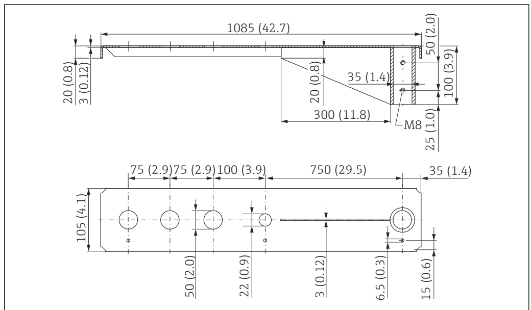
33 Abmessungen. Maßeinheit mm (in)
