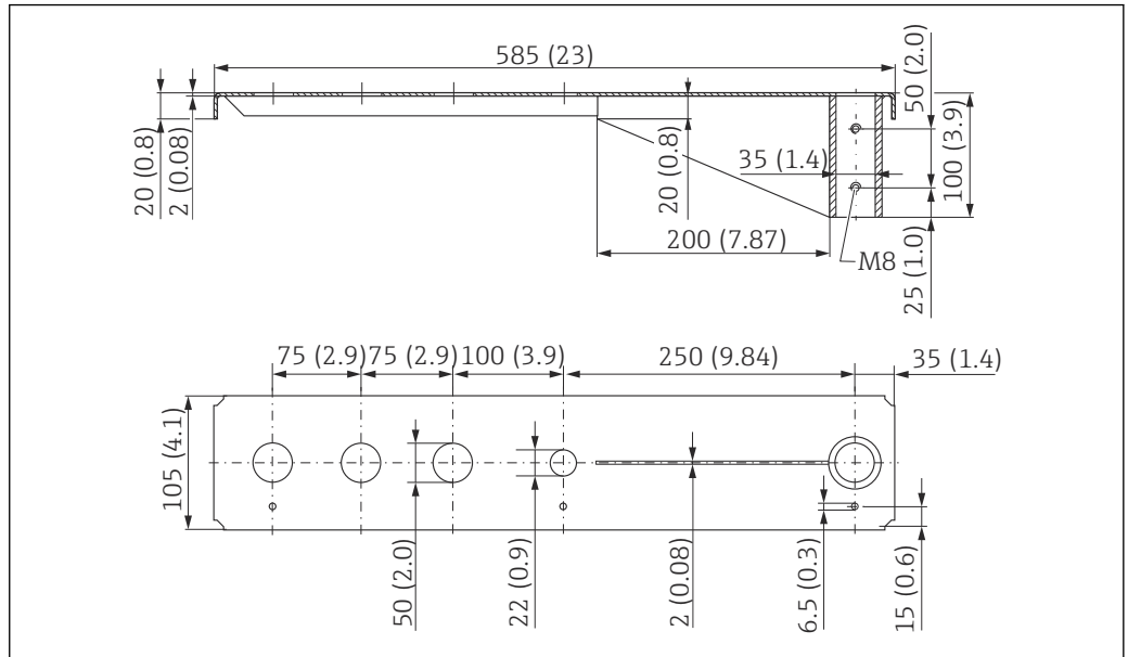
32 Abmessungen. Maßeinheit mm (in)
