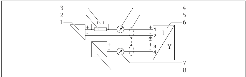
図 7 ブロック図、2 線式：4～20 mA HART、4～20 mA
