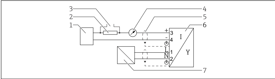
図 11 ブロック図、4 線式：4～20 mA HART（90～253 V AC ）
