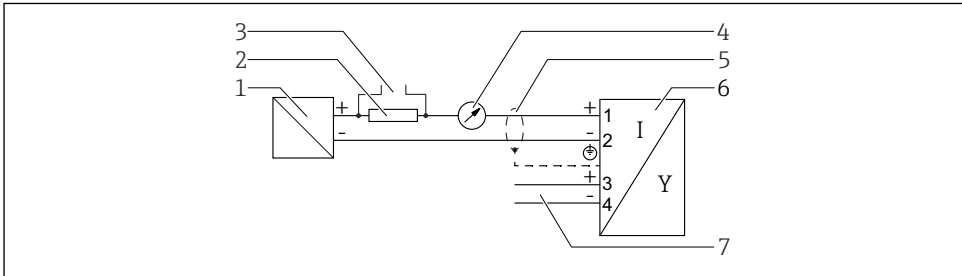
図 5 ブロック図、2 線式：4～20 mA HART、スイッチ出力
