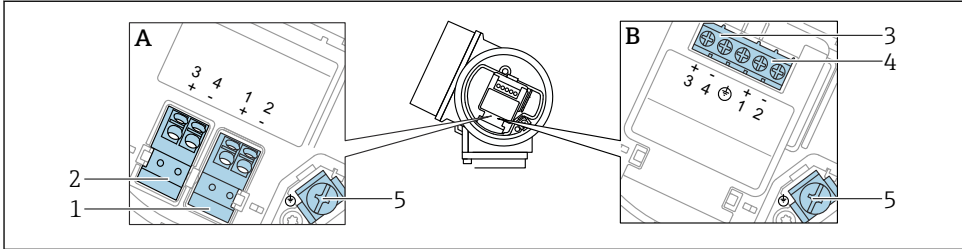
図 4 端子の割当て、2 線式：4～20 mA HART、スイッチ出力
