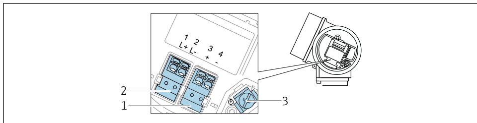
8 端子の割当て、4線式：4～20 mA HART (10.4～48 V DC )
