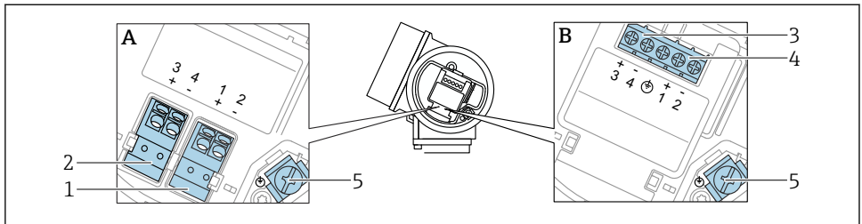
図 6 端子の割当て、2 線式：4～20 mA HART、4～20 mA
