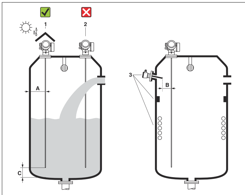
図 1 Levelflex の設置条件
