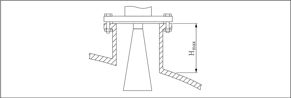
2 Kaulusputken korkeus torviantennille (FMR51)
