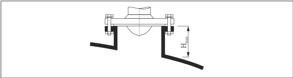
3 Stoshöjd för hornantenn, försänkt montering (FMR52)
