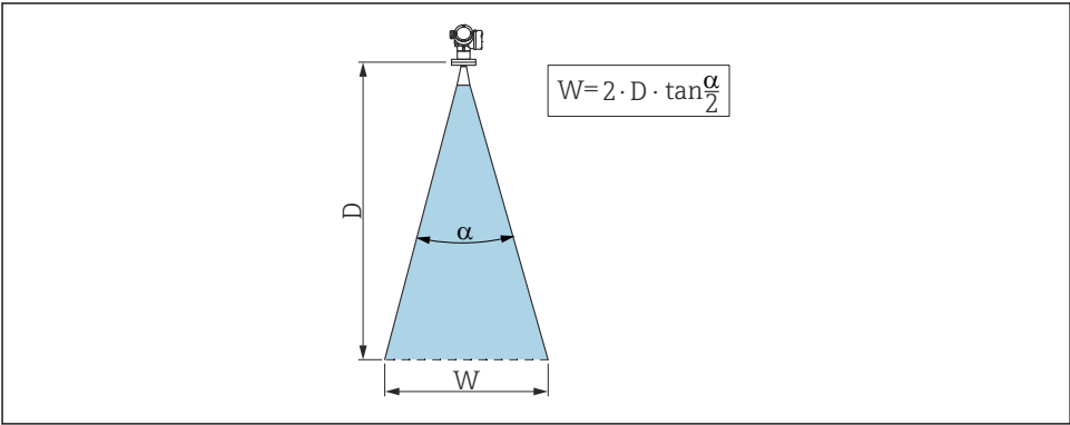
1 Rapporto tra angolo di emissione \alpha , distanza D e diametro del lobo di emissione W
