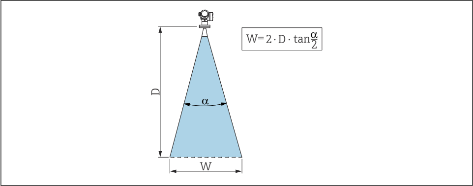
1 Vztah mezi vyzařovacím úhlem \alpha , vzdáleností D a průměrem paprsku W
