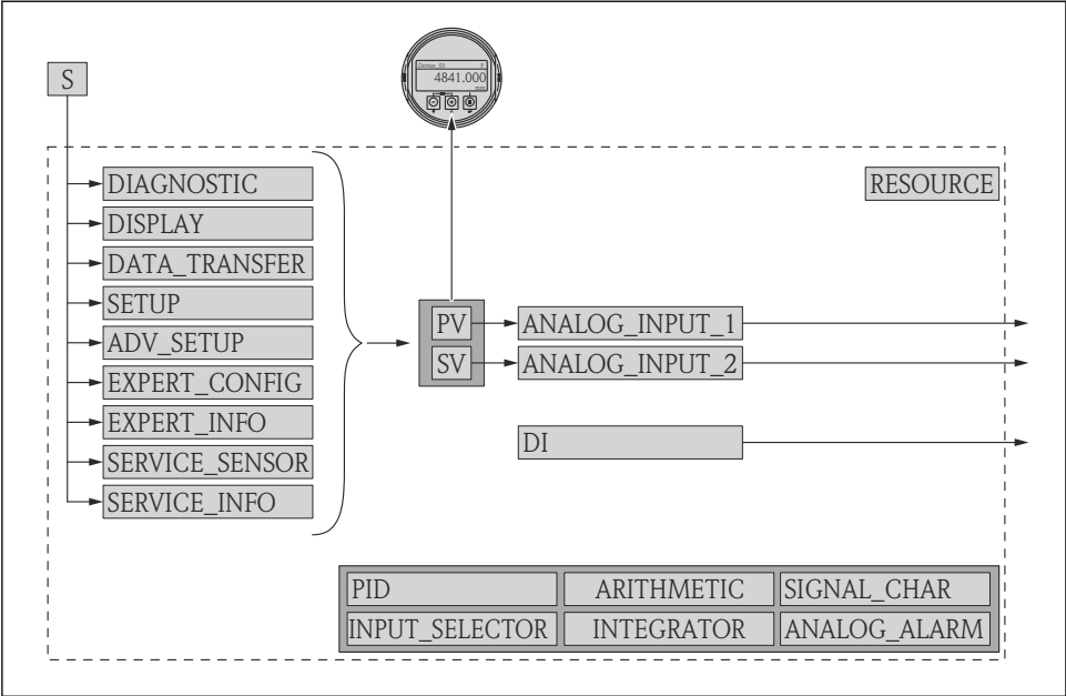
10 Konfigurace bloků při dodání zařízení
