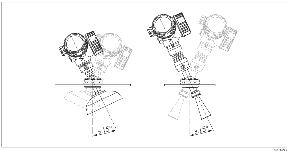
6 Micropilot FMR57 med innrettingsenhet
