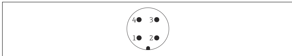
5 Přirazení kontaktů konektoru M12
