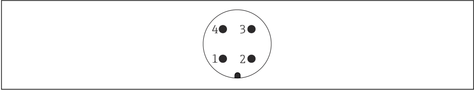
図 5 M12 プラグのピン割当て
