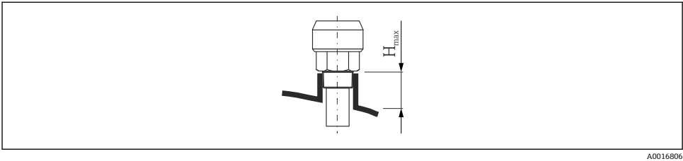
2 被覆ホーンアンテナ（FMR50）のノズル高、 H_{\max} = 60 mm (2.36 in)
