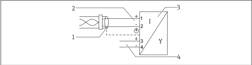
図 4 ブロック図：PROFIBUS PA / FOUNDATION フィールドバス
