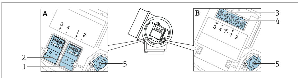
図 3 端子の割当て PROFIBUS PA / FOUNDATION フィールドバス
