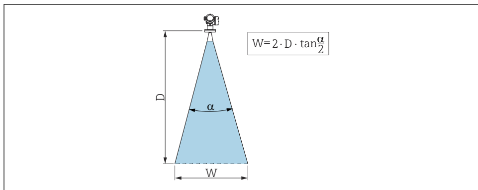
図 1 放射角 \alpha 、距離 D 、ビーム幅 W の関係
