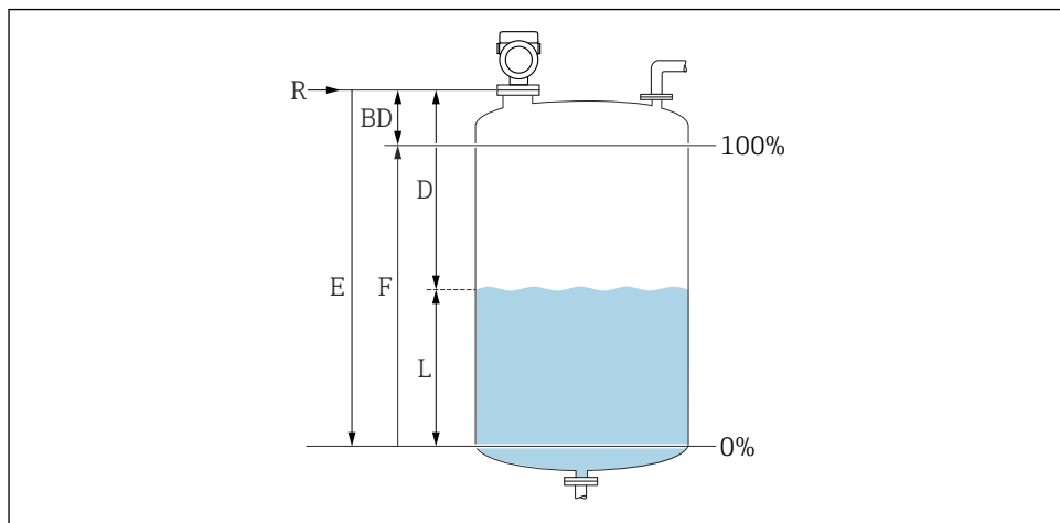
16 Параметры конфигурации для измерения уровня жидкости
