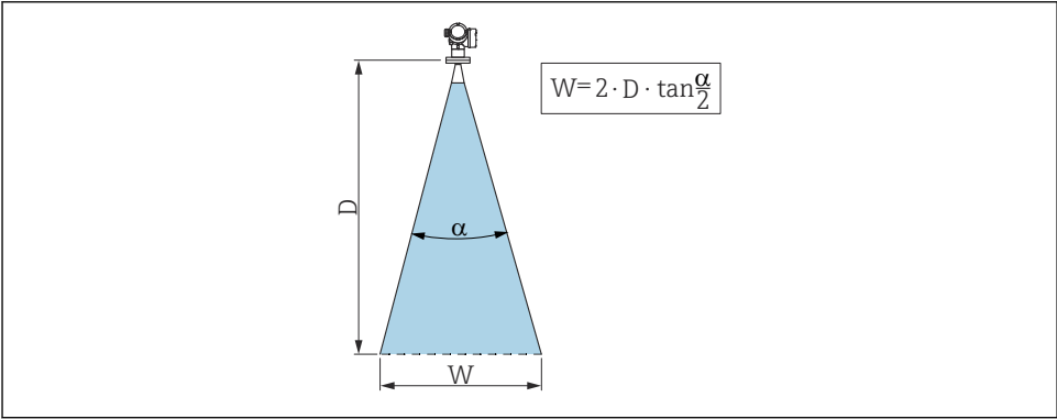
1 Взаимосвязь между углом расхождения луча α, расстоянием D и диаметром луча W
