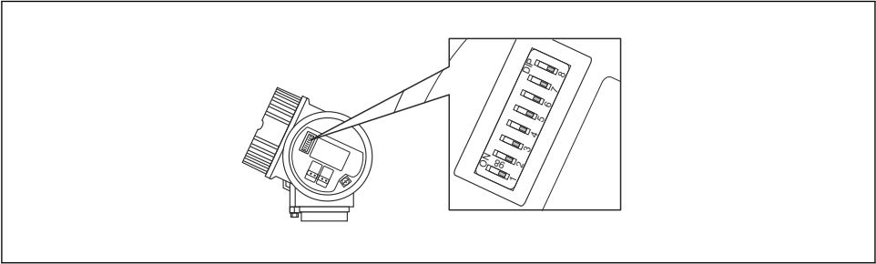
9 Переключатель адресов в клеммном отсеке
