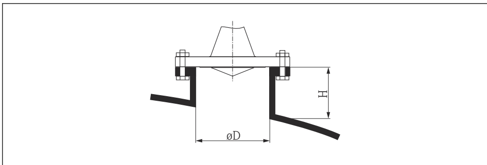
2 Dysediameter og højde for hornantenner med glat flange
