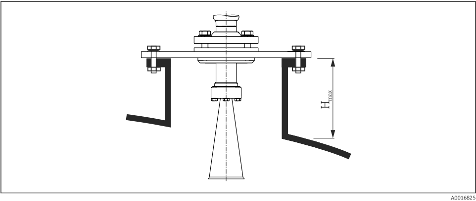
4 Stosens höjd för hornantenn (FMR57)
