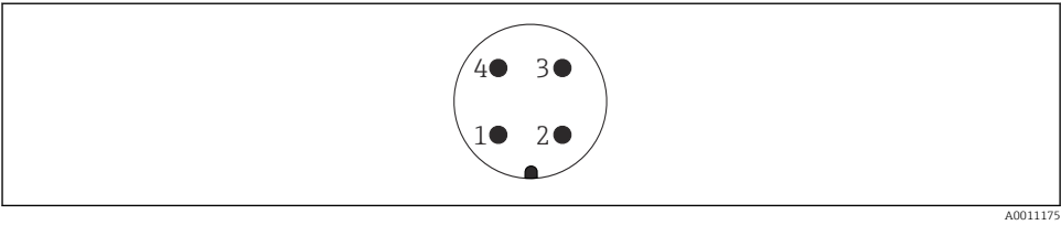
10 Razpored pinov v konektorju M12
