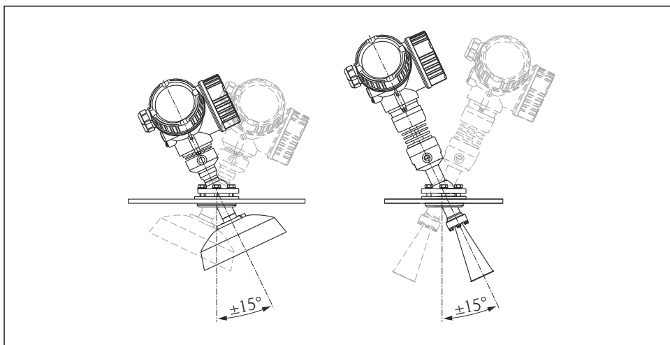
6 Micropilot FMR57 s pripravo za poravnavanje
