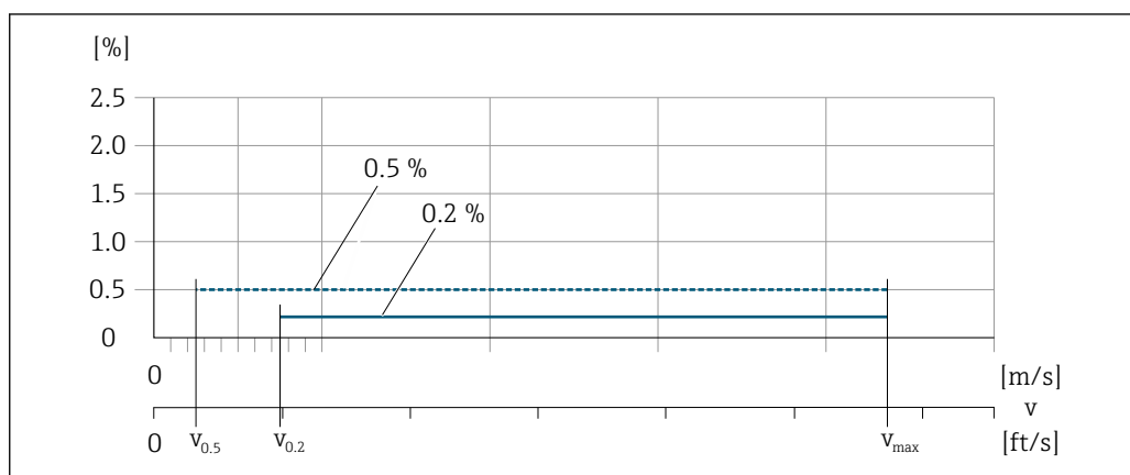
図 23 フラットスペック (%) o.r.
