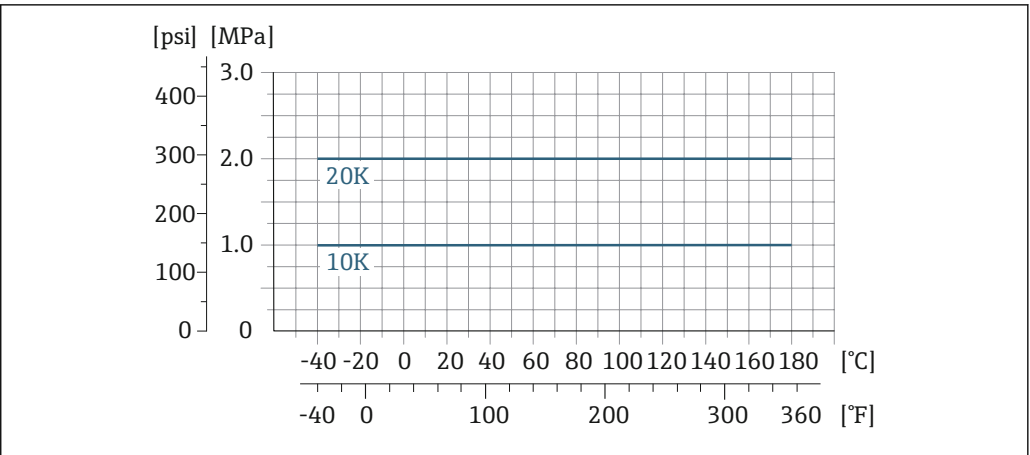
33 プロセス接続材質 : ステンレス SUS F316L 相当 ; 炭素鋼 S235JRG2/HII
