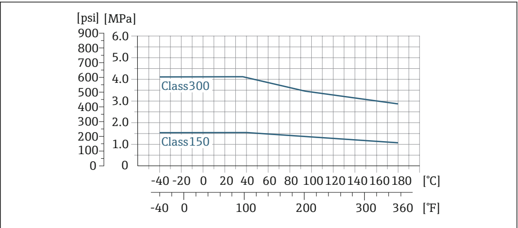
32 プロセス接続材質 : ステンレス SUS F316L 相当
