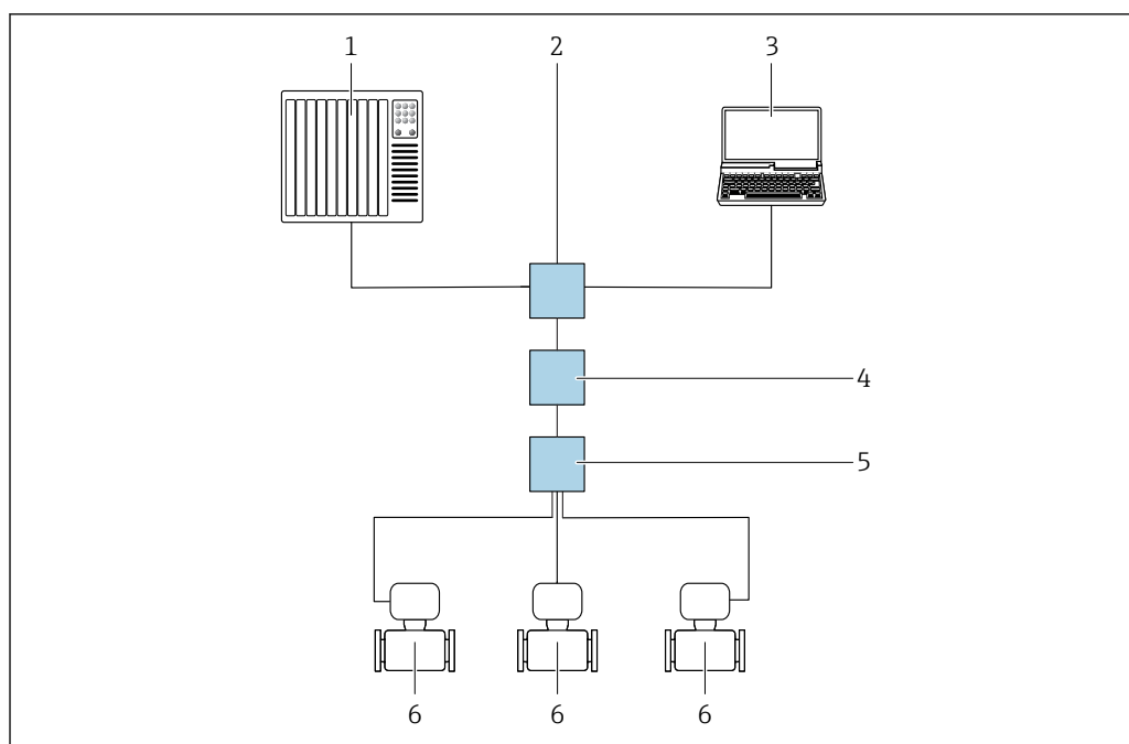
図 57 APL ネットワーク経由のリモート操作オプション
