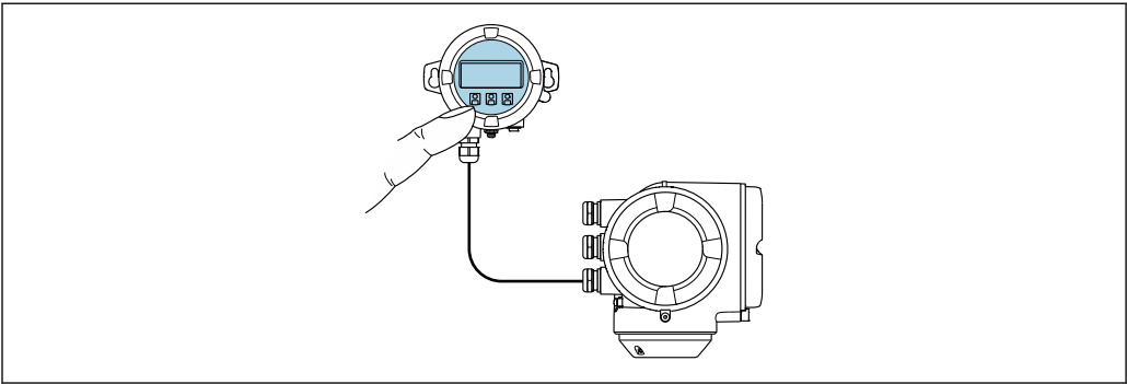
46 分離型ディスプレイと操作モジュール DKX001 を介した操作
