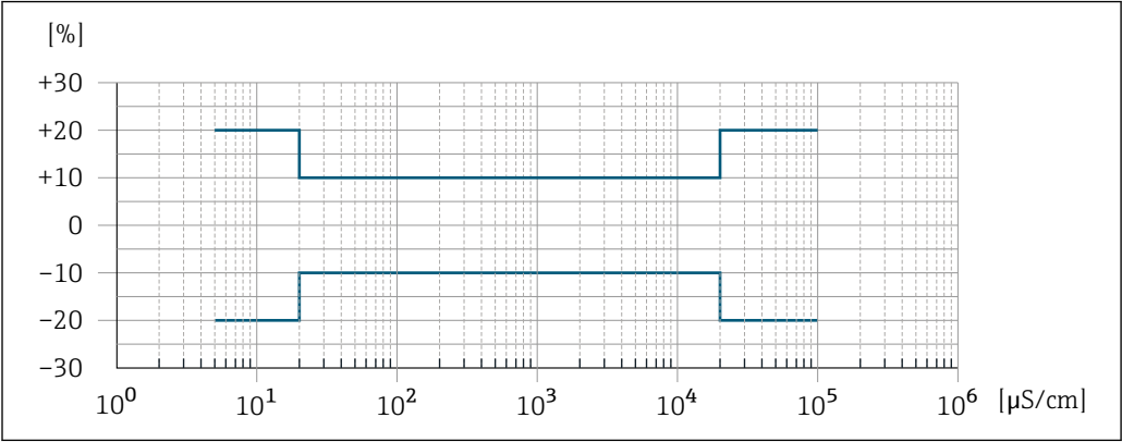
図 24 測定誤差（標準）
