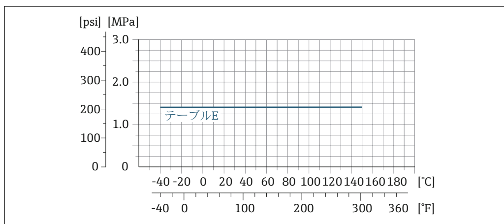
図 34 プロセス接続材質：炭素鋼 A105/S235JRG2/S275JR
