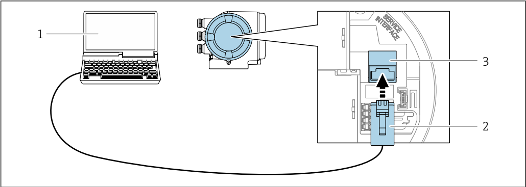
■ 58 サービスインターフェイス（CDI-RJ45）経由の接続
