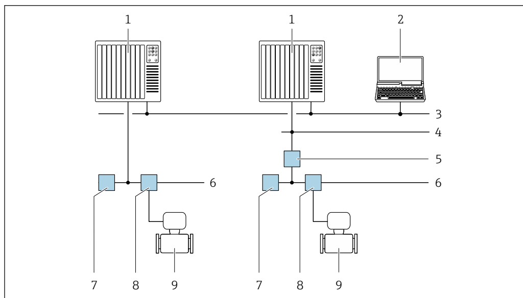
図 49 FOUNDATION フィールドバスネットワークを介したリモート操作のオプション
