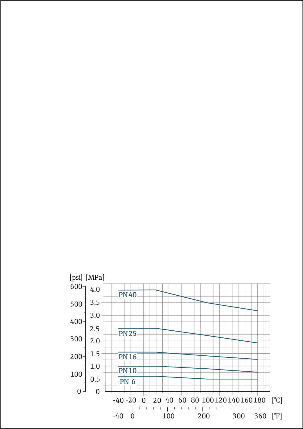
30 プロセス接続材質：ステンレス 1.4571
