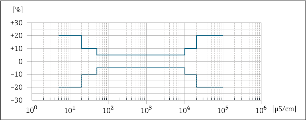
図 25 測定誤差（オプション：「校正された導電率測定」のオーダーコード、オプション CW）
