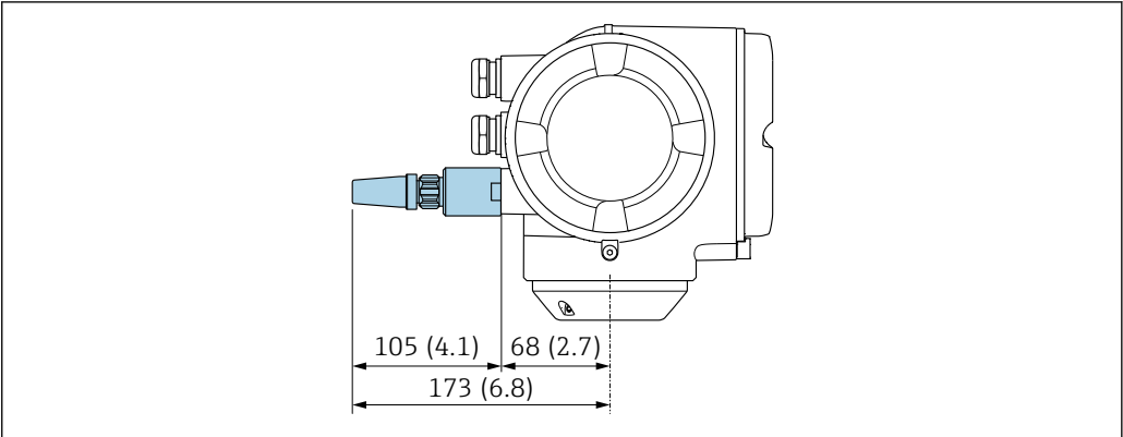
42 単位 mm (in)
