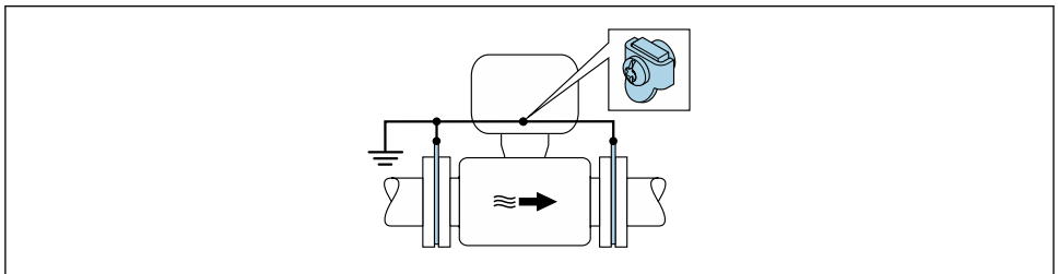
5 Compensation de potentiel via la borne de terre et les disques de mise à la terre ( PE = P_{FL} = P_M )
