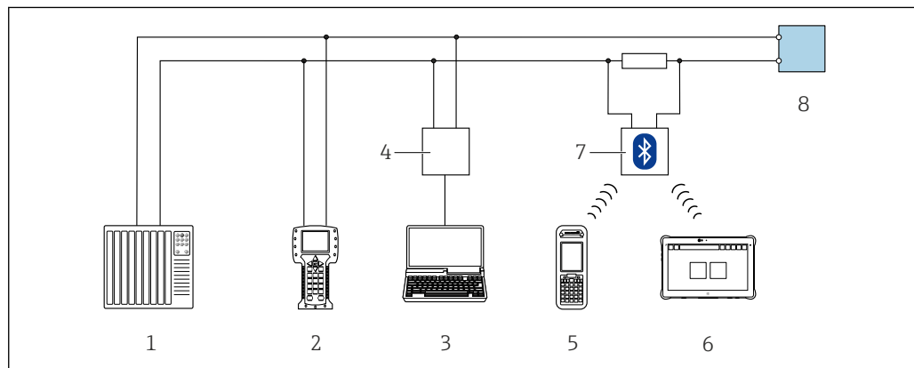
図 46 HART プロトコル経由のリモート操作用オプション（アクティブ）
