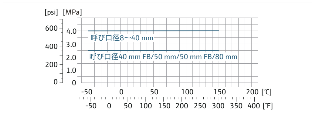
図 30 接続部材質 Grade 2 チタン
