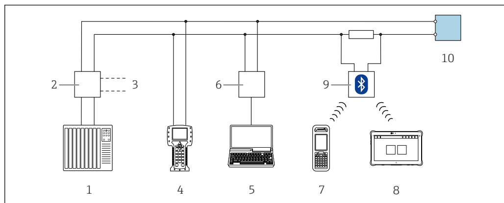
図 47 HART プロトコル経由のリモート操作用オプション（パッシブ）
