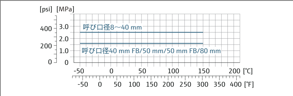
図 28 フランジ材質 Grade 2 チタン
