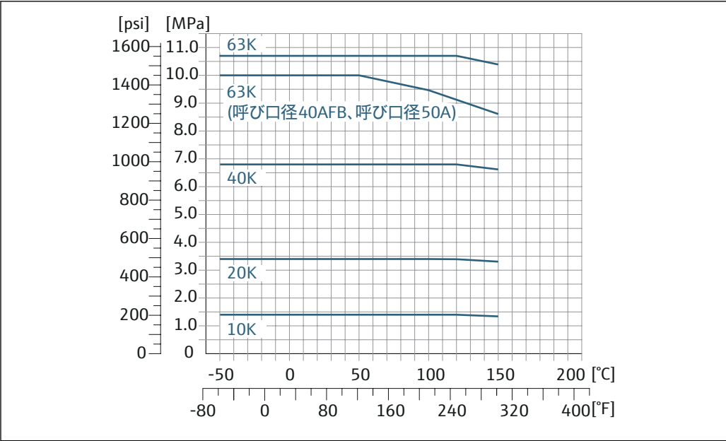
図 27 フランジ材質 1.4301 (SUS 304 相当)。接液部：チタン
