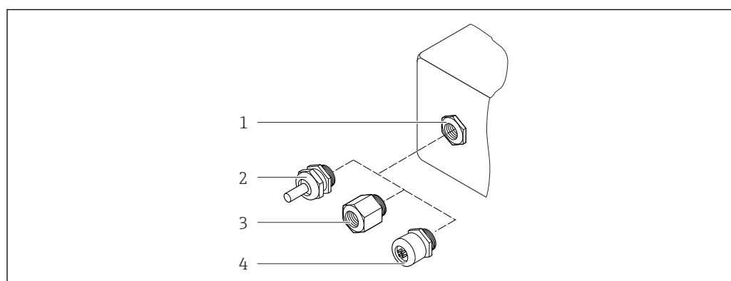
図 43 可能な電線管接続口/ケーブルグラウンド
