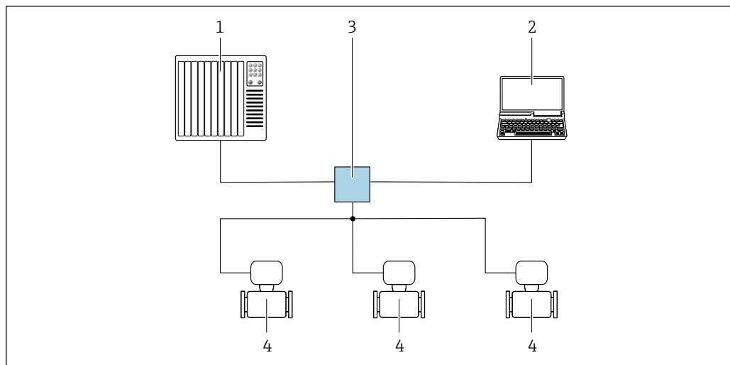
図 54 PROFINET ネットワーク経由のリモート操作オプション：スター型トポロジー
