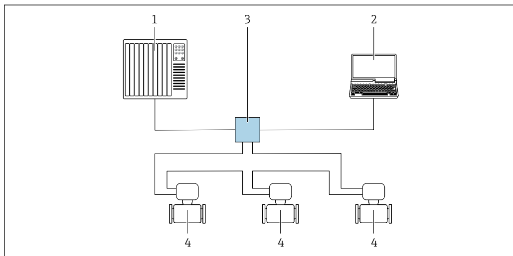
図 55 PROFINET ネットワーク経由のリモート操作オプション：リング型トポロジー
