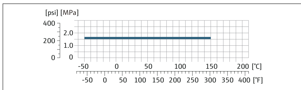
図 32 接続部材質 Grade 2 チタン
