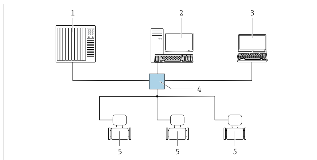
図 52 EtherNet/IP ネットワーク経由のリモート操作オプション：スター型トポロジー
