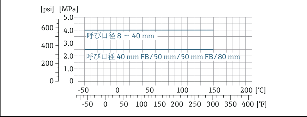
図 29 接続部材質 Grade 2 チタン
