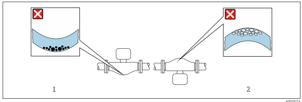
24 Position du capteur avec tube de mesure coudé
