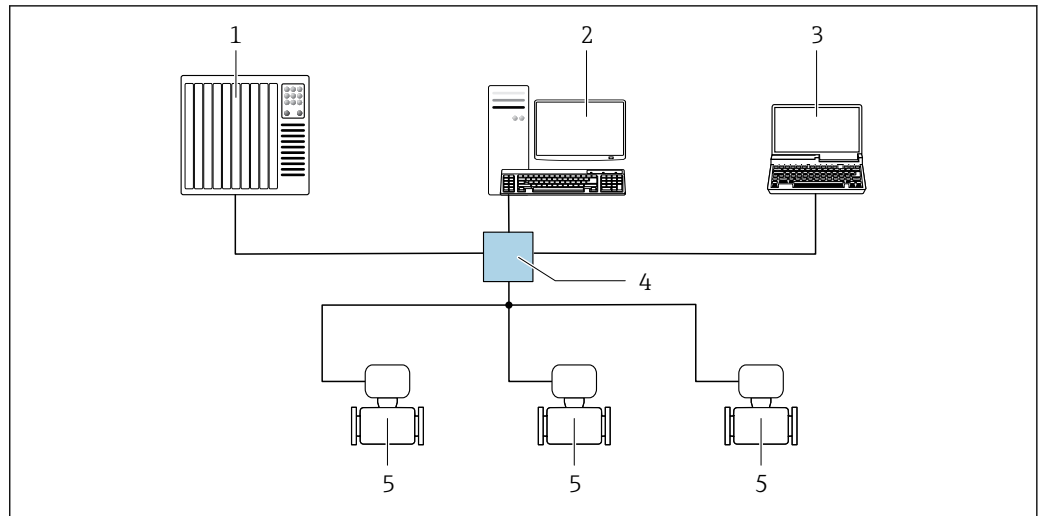
55 Options pour la configuration à distance via le réseau EtherNet/IP : topologie en étoile
