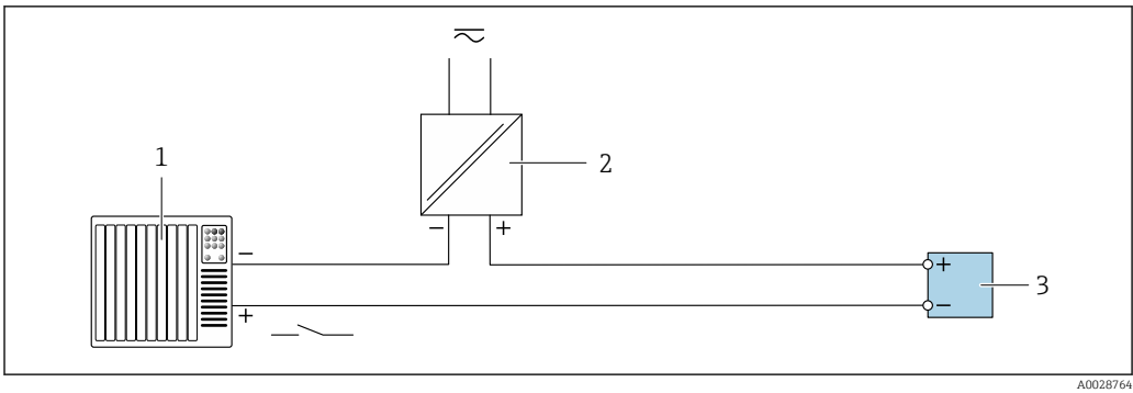
21 Exemple de raccordement pour l'entrée état
