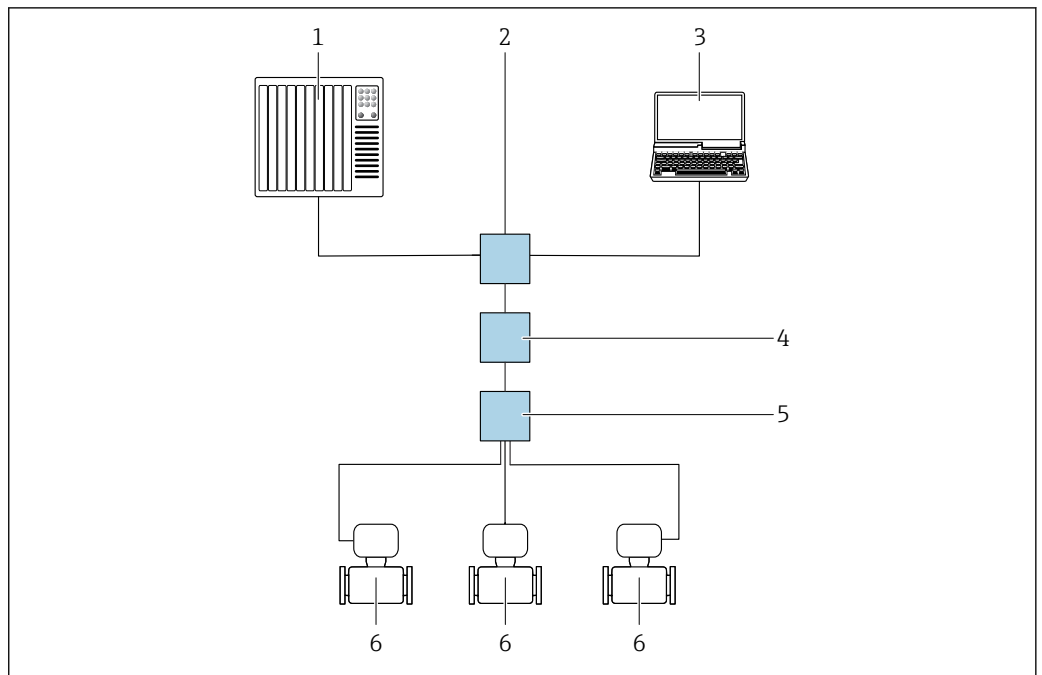
59 Options pour configuration à distance via réseau APL
