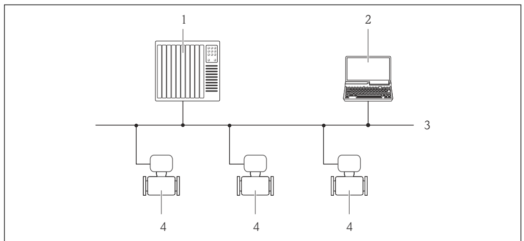
52 Possibilités de configuration à distance via réseau PROFIBUS DP
