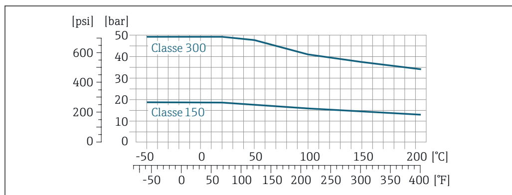
32 Con flangia in 1.4301 (304); parti bagnate: zirconio 702, tantalio
