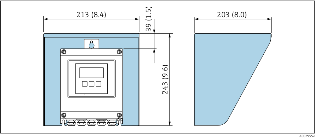
28 Tettuccio di protezione dalle intemperie per Proline 500 – digitale; unità ingegneristica mm (in)
