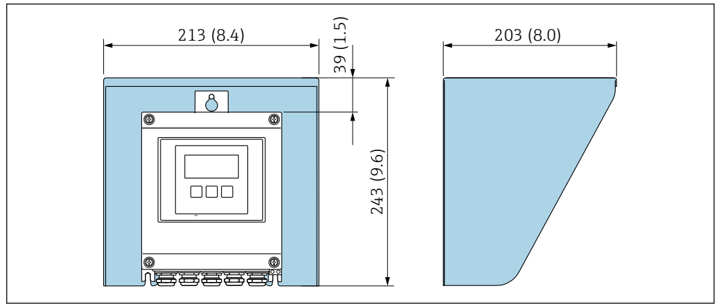
35 Tettuccio di protezione dalle intemperie per Proline 500 – digitale; unità ingegneristica mm (in)
