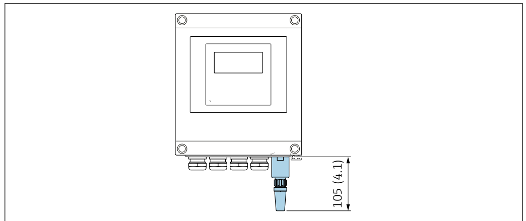
37 Unità ingegneristica, mm (in)
