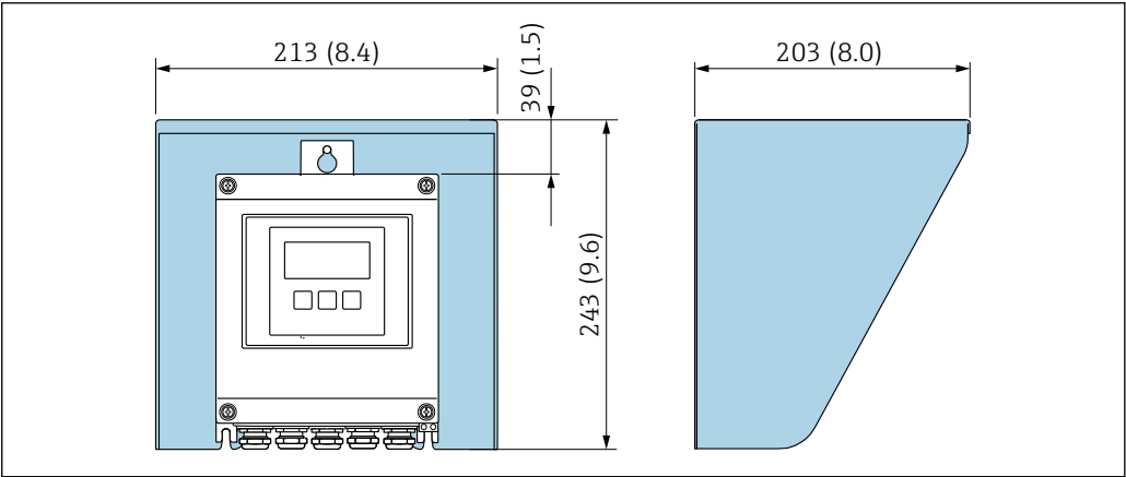
41 Tettuccio di protezione dalle intemperie per Proline 500 – digitale; unità ingegneristica mm (in)
