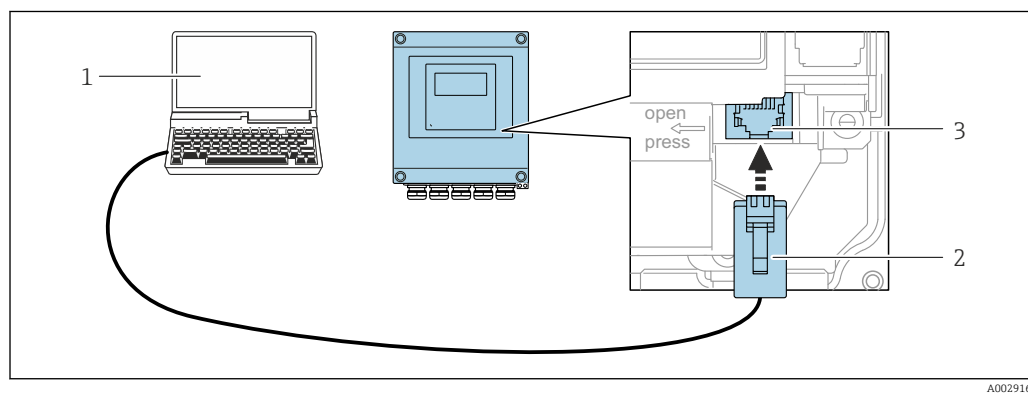
60 Connessione mediante interfaccia service (CDI-RJ45)
