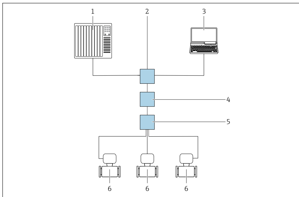
60 Options pour configuration à distance via réseau APL
