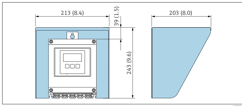
36 Capot de protection climatique pour Proline 500 – numérique ; unité de mesure mm (in)
