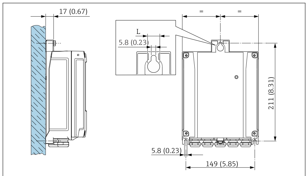
25 Unité de mesure mm (in)
