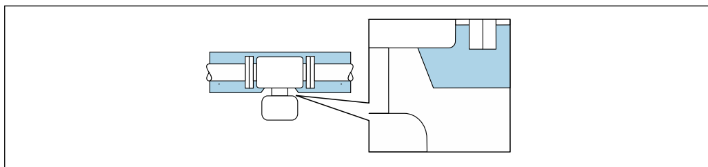
34 Isolation thermique avec tube prolongateur non isolé
