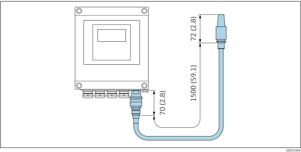
39 Unité de mesure mm (in)
