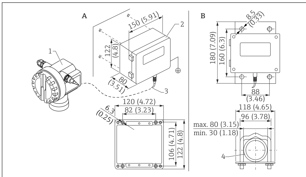
30 Indicador remoto. Unidad de medida mm (in)
