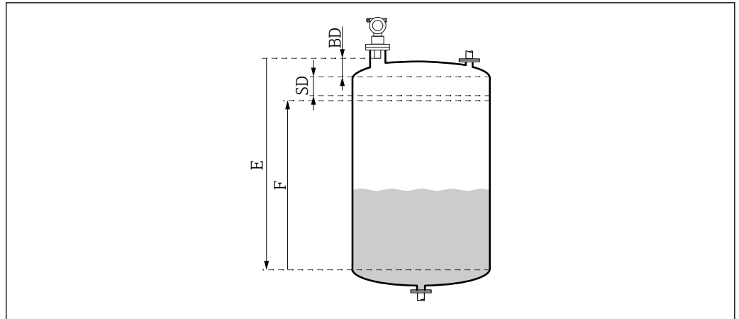
14 Parámetros para el funcionamiento correcto del equipo
