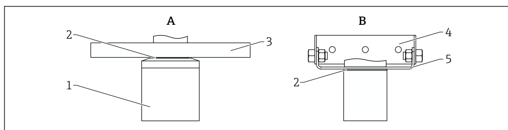
22 A: brida; B: soporte de montaje
