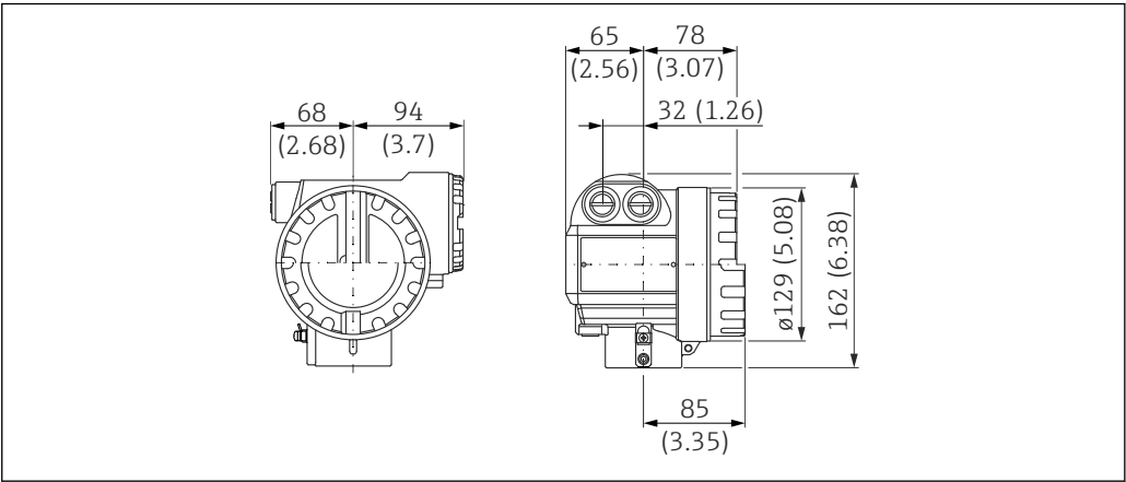
17 Medidas de la caja T12. Unidad de medida mm (in)
