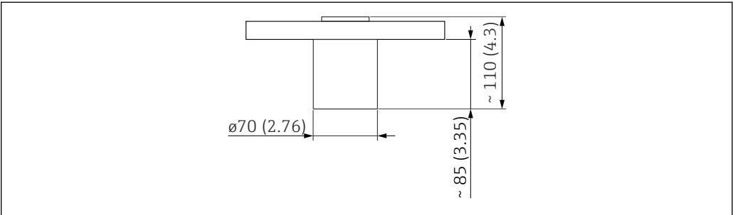
18 Medidas del sensor . Unidad de medida mm (in)
