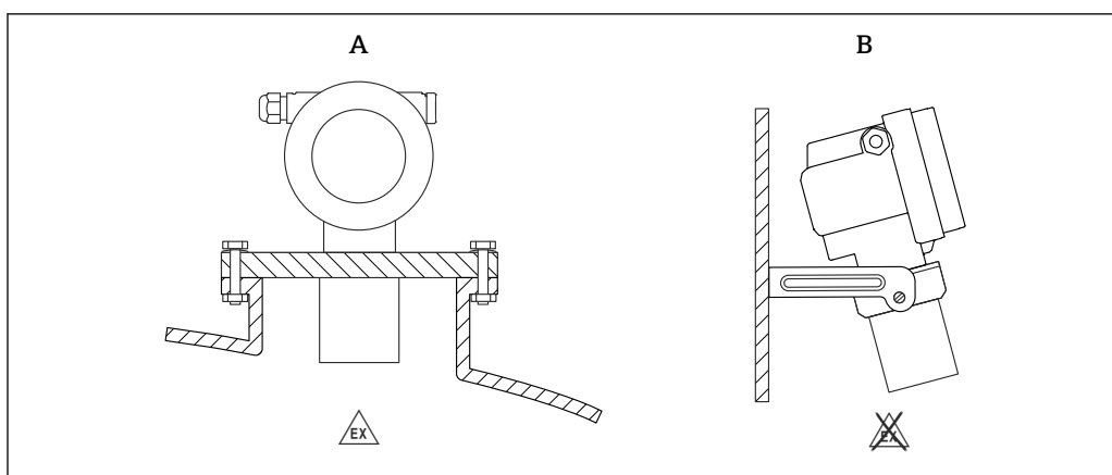
12 Ejemplos de montaje
