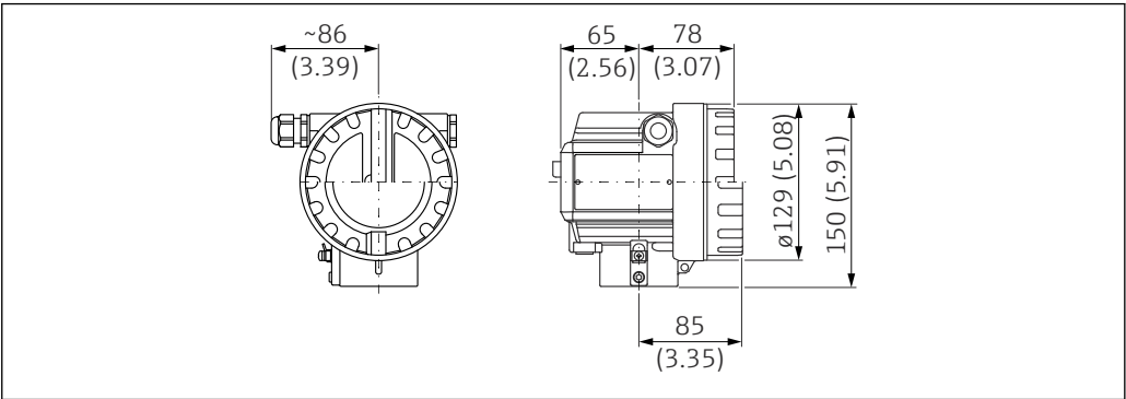
16 Medidas de la caja F12. Unidad de medida mm (in)
