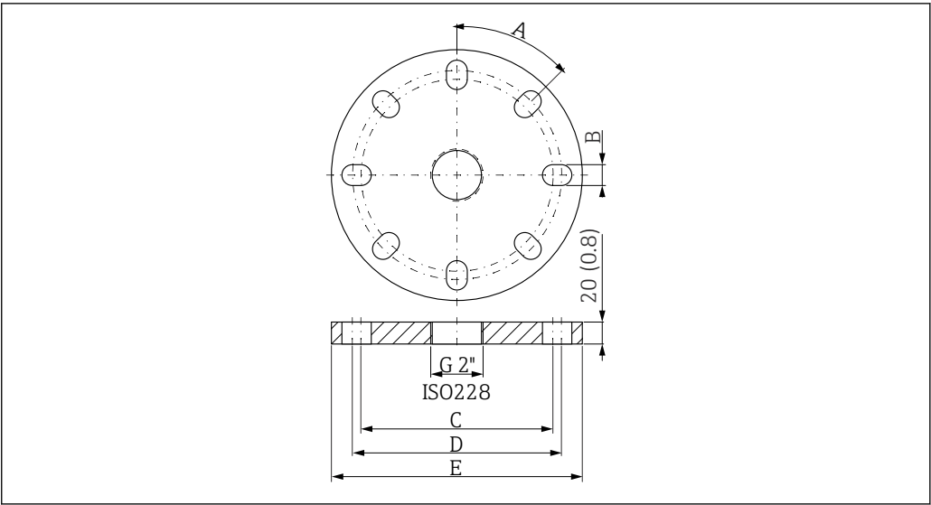
21 Brida. Unidad de medida mm (in)
