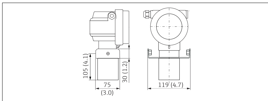
19 Medidas con soporte de montaje . Unidad de medida mm (in)
