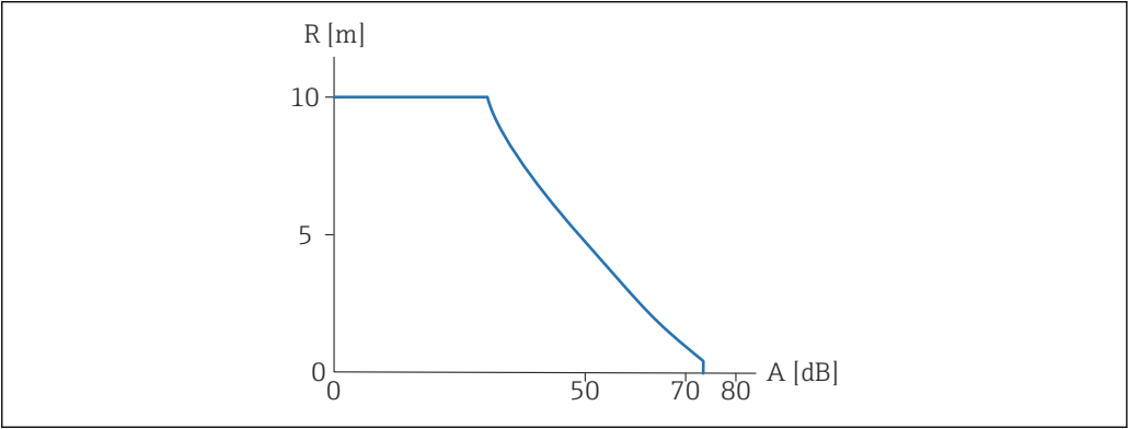
4 Gráfico de alcance
