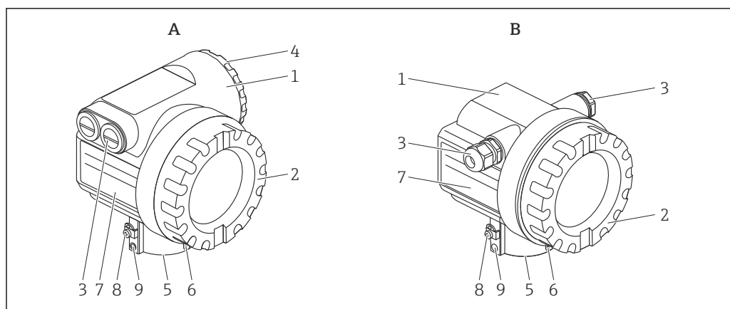
23 A: caja T12; B: caja F12
