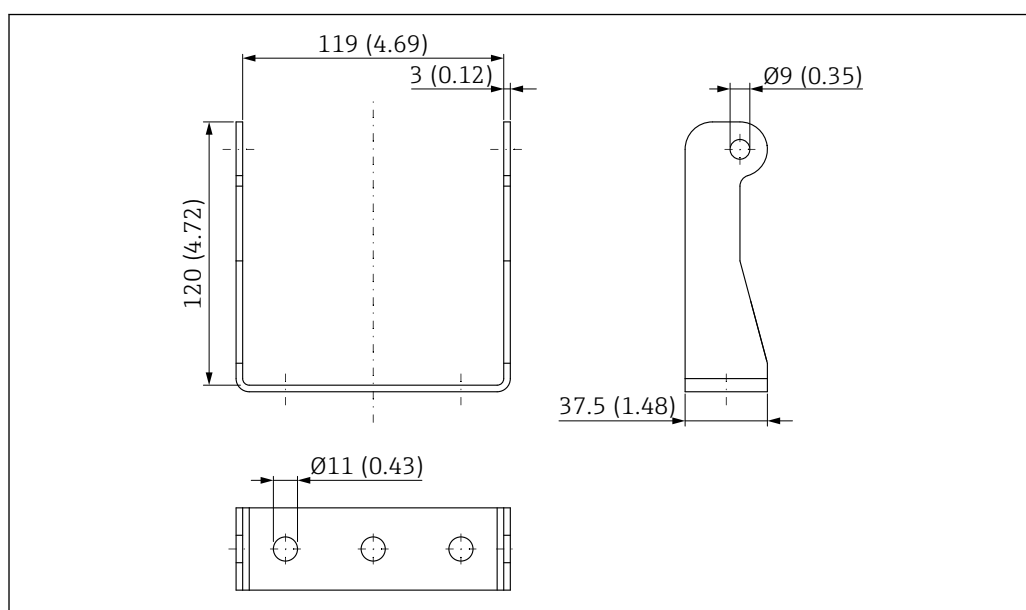
20 Soporte de montaje. Unidad de medida mm (in)
