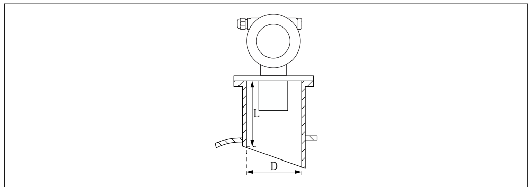
15 Definición de la longitud de la tubuladura L y del diámetro de la tubuladura D
