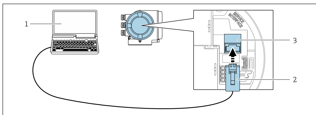
29 Conexão através de Interface de operação (CDI-RJ45)
