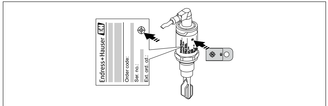
図 29 ハウジングに対するテストマグネットの位置
