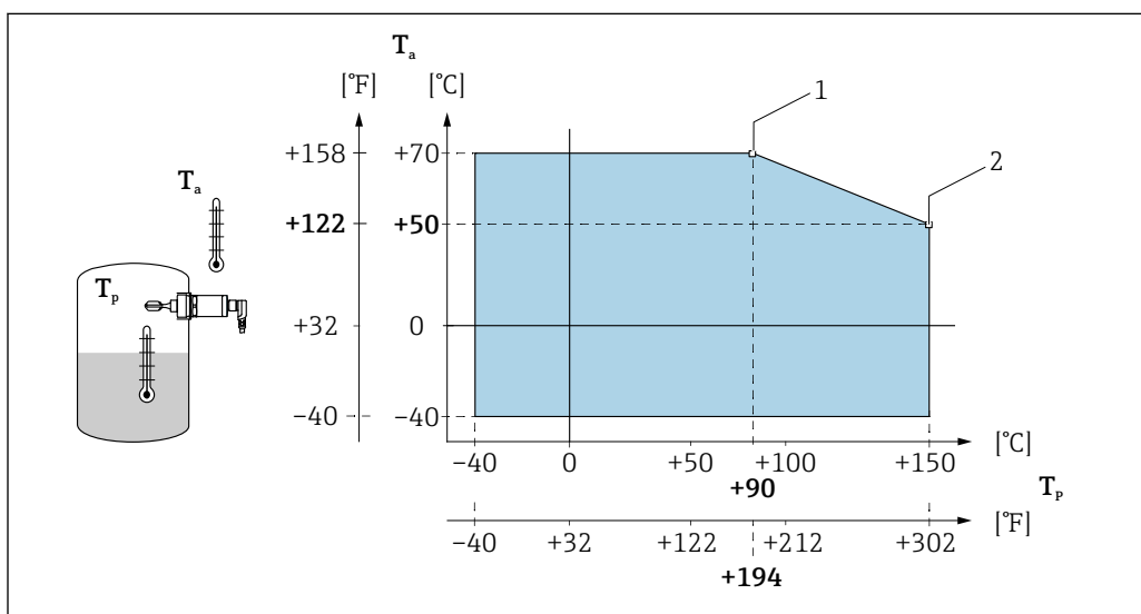
図 12 ディレーティング曲線 : 150 °C (302 °F)
