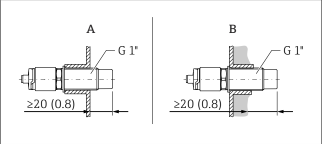
2 Maßeinheit: mm (in) A Standardeinbau mit Gewindestutzen G 1" nach außen B Bei Ansatzbildung an der Silowand mit Gewindestutzen G 1" nach innen
