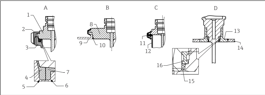
图 5 保证卫生合规的安装指南（取决于仪表选型）
