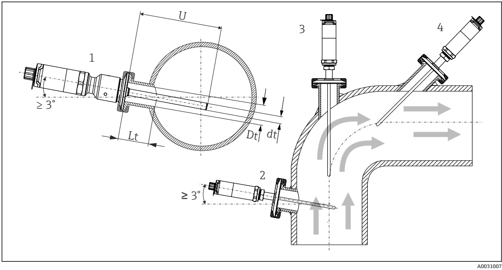
图 3 在过程中的允许安装位置 1、2 安装方向与介质流向垂直，为了确保自排空，倾斜安装角度不得小于 3° 3 安装在管道弯头位置处 4 倾斜安装在小标称口径管道中 U 插深
