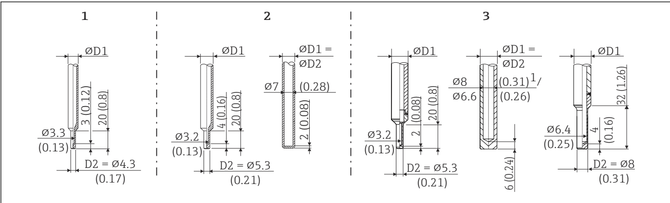
图 11 保护套管末端类型（缩径型、直管型、锥管型）
