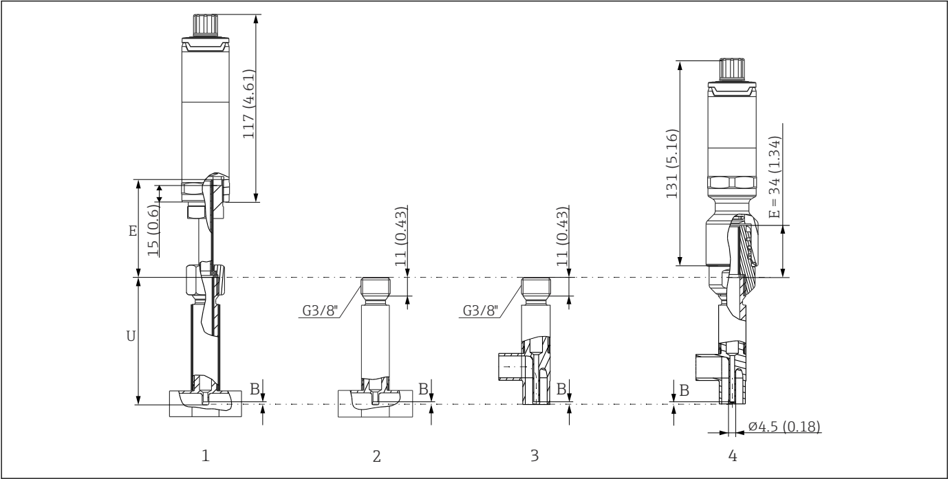
温度计，带 T-piece 或直角弯头保护套管
