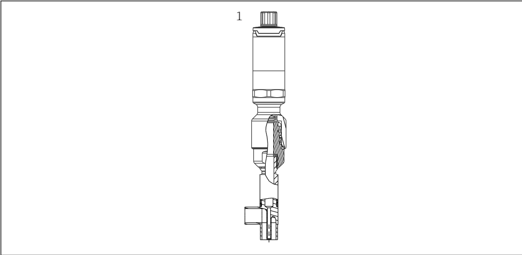
图 4 在小标称口径管道中安装的温度计的过程连接
