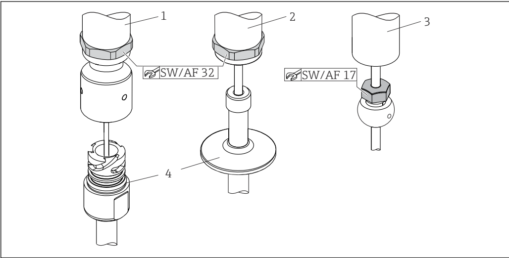
图 2 紧凑型温度计的安装过程
