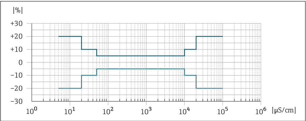
26 测量误差 (可选: 订购选项“电导率测量标定”, 选型代号 CW)
