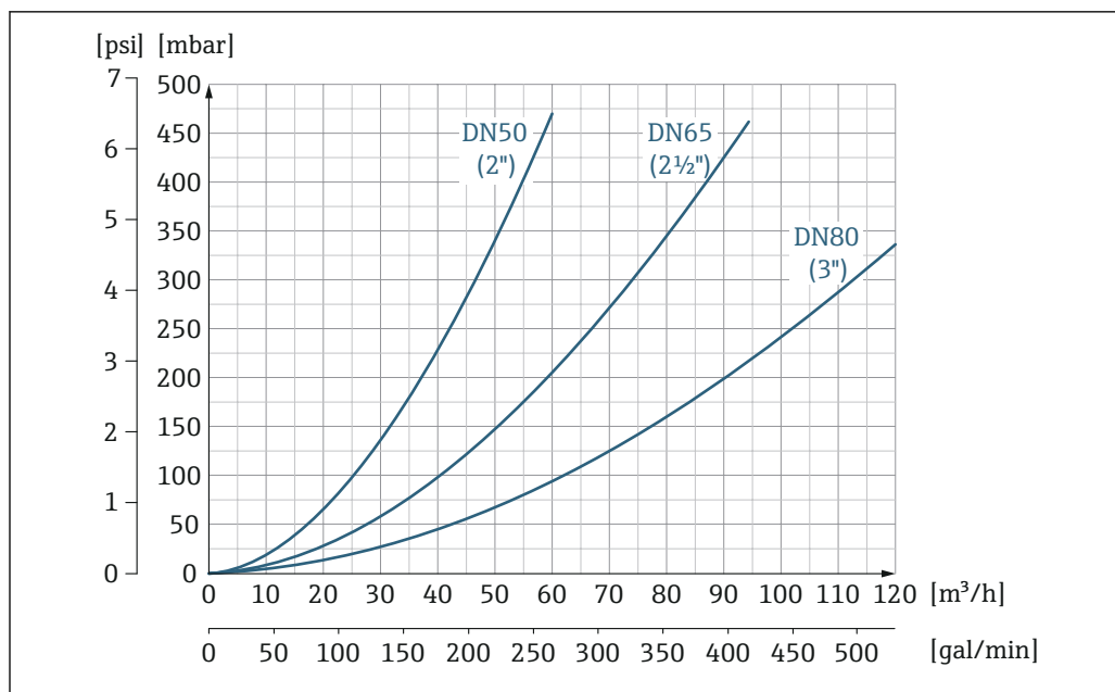
图 42 压损：适用口径 DN 50...80 (2...3"); 订购选项“设计”，选型代号 C “固定法兰，缩径测量管，无前后直管段长度要求”
