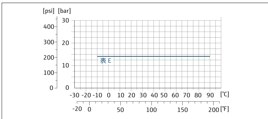
图 39 过程连接材质: 碳钢
