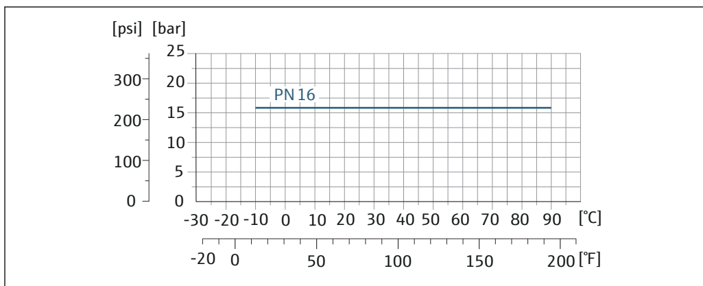
图 40 过程连接材质: 碳钢
