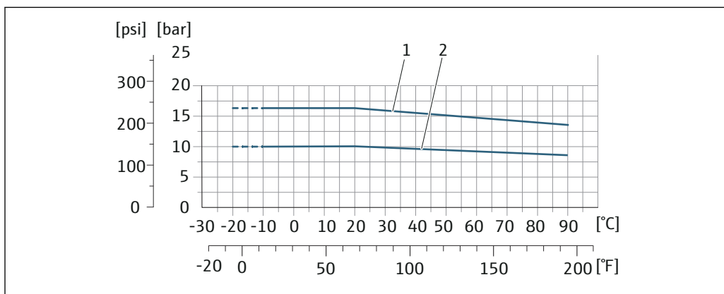
图 41 过程连接材质: 不锈钢 (-20 °C (-4 °F)) ; 碳钢 (-10 °C (14 °F))
