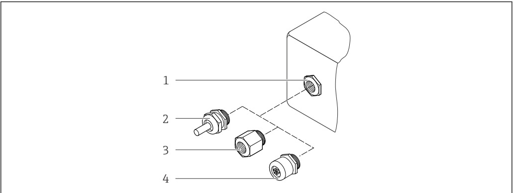
图 57 允许的电缆入口/缆塞
