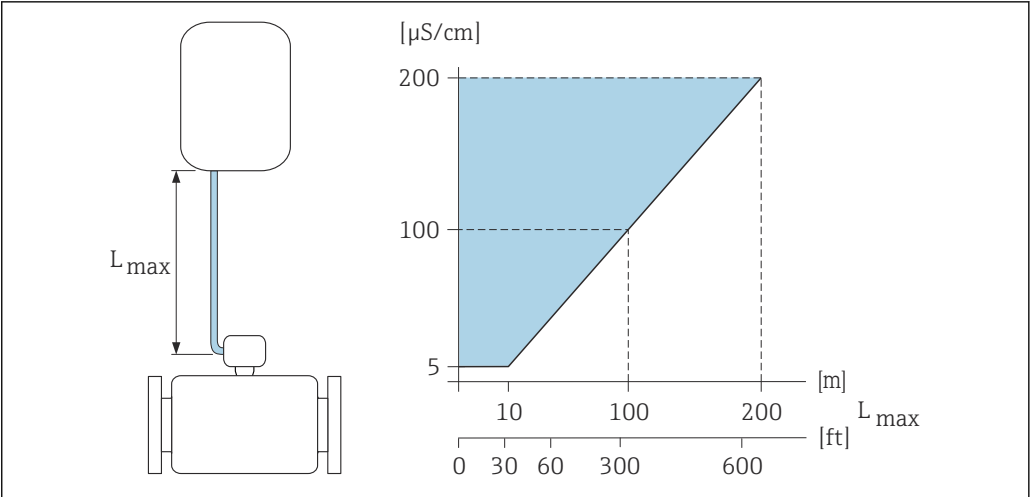
27 允许连接电缆长度 彩色区域 = 允许电缆长度范围 L_{\max} = 连接电缆长度 ([m] ([ft]) ) [\mu\text{S/cm}] = 介质电导率
