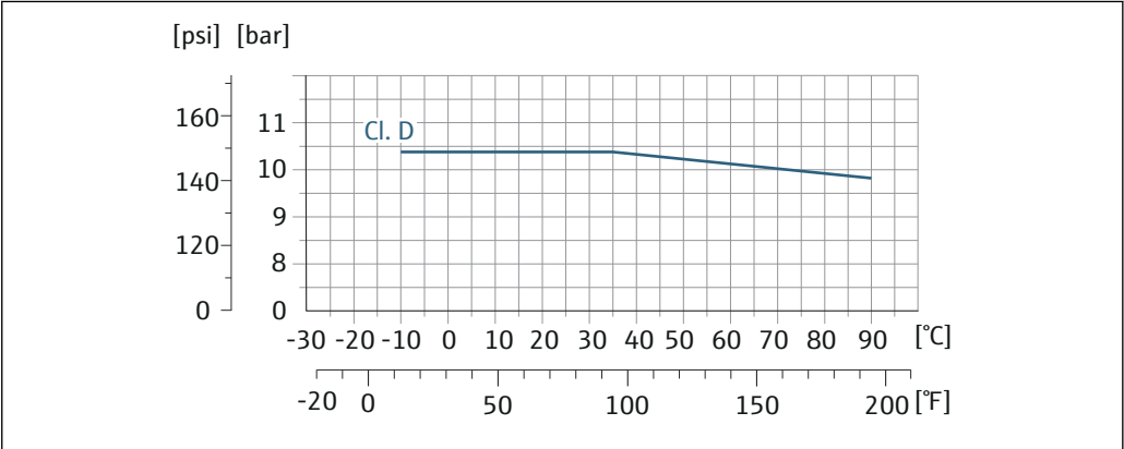
38 过程连接材质：碳钢
