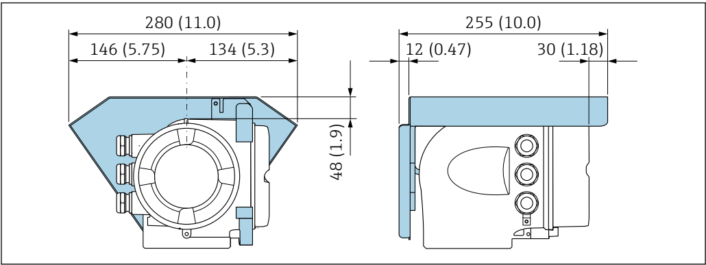
图 33 Proline 500（模拟）变送器的防护罩的外形尺寸图；单位：mm (in)
