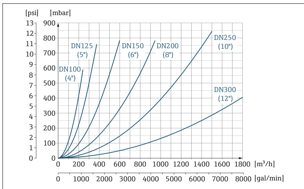
图 43 压损：适用口径 DN 100...300 (4...12"); 订购选项“设计”，选型代号 C “固定法兰，缩径测量管，无前后直管段长度要求”
