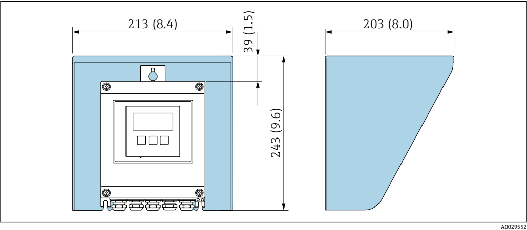
45 Proline 500 (数字) 变送器的防护罩的外形尺寸图; 单位: mm (in)
