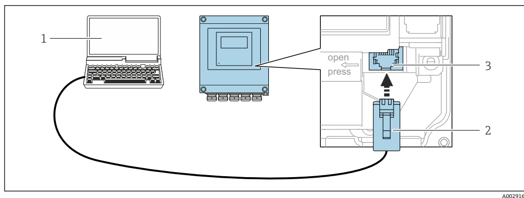
图 70 通过服务接口 (CDI-RJ45) 连接
