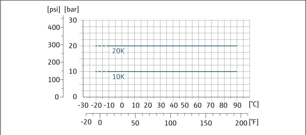
37 过程连接材质：不锈钢（-20 °C (-4 °F)）；碳钢（-10 °C (14 °F)）
