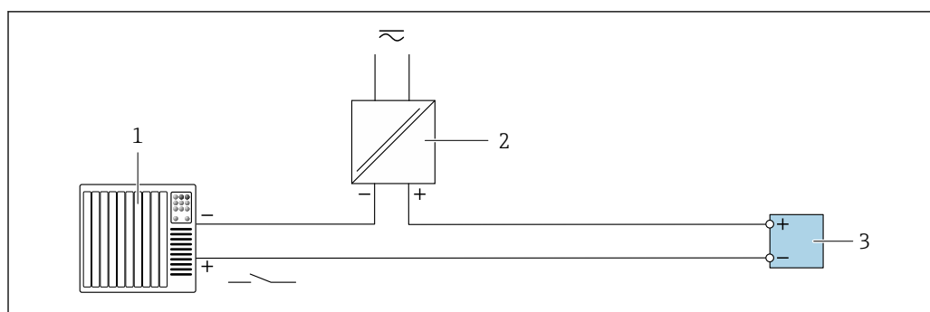
21 接线实例：状态输入
