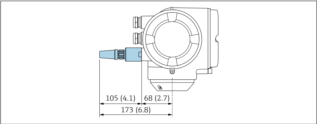
图 47 单位: mm (in)
