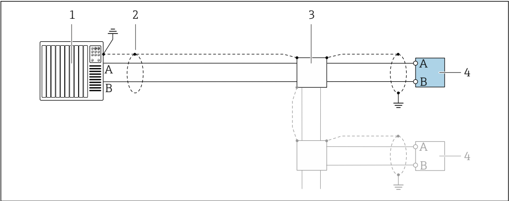
6 接线实例：PROFIBUS DP，非危险区和防爆 2 区/ Div. 2 防爆场合
