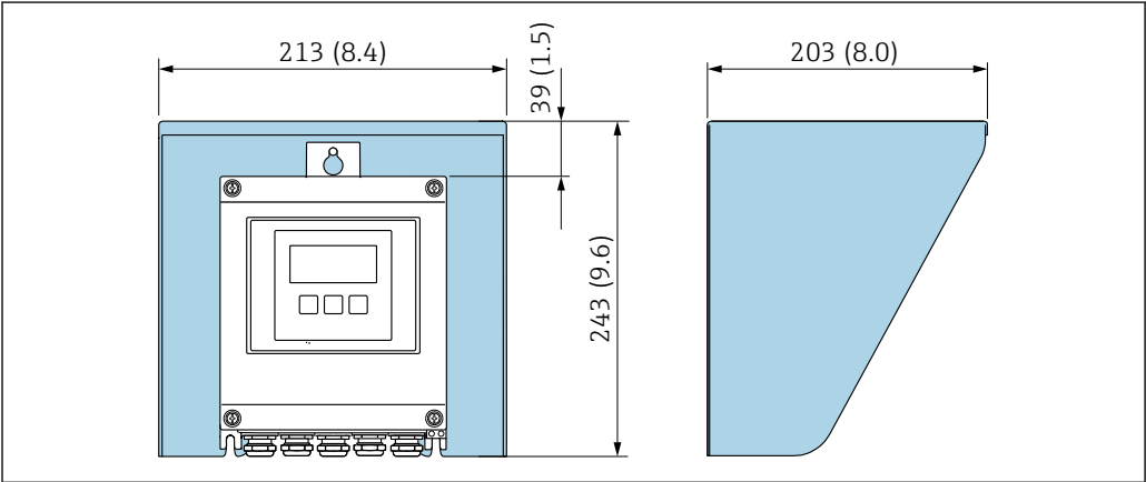
图 49 Proline 500 (数字) 变送器的防护罩的外形尺寸图; 单位: mm (in)
