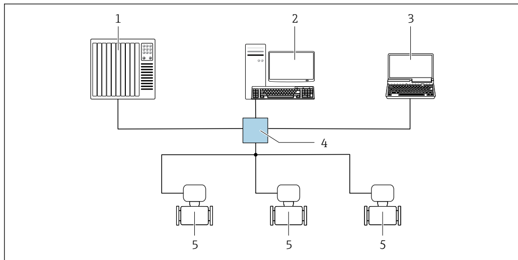
图 63 通过 EtherNet/IP 网络进行远程操作：星形拓扑结构
