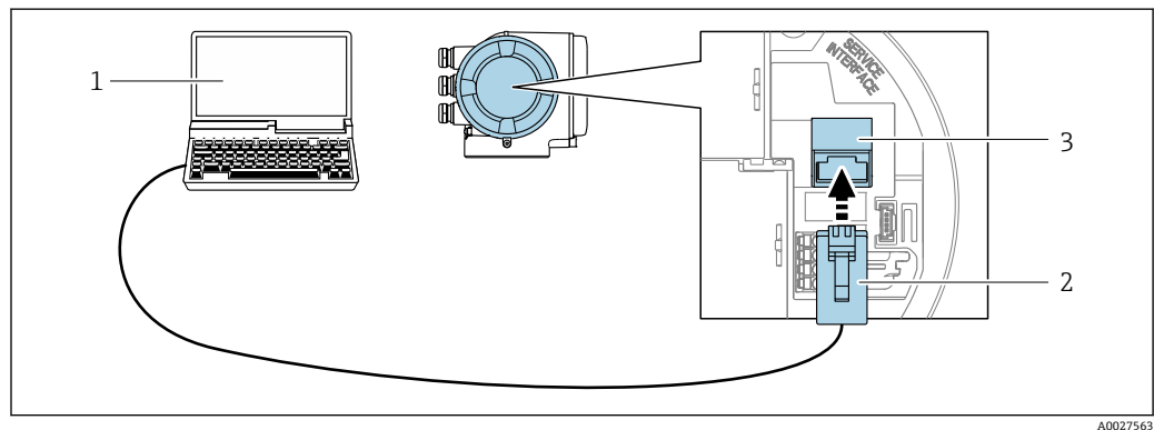
图 69 通过服务接口 (CDI-RJ45) 连接
