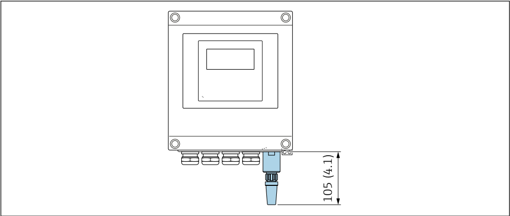
45 单位：mm (in)
