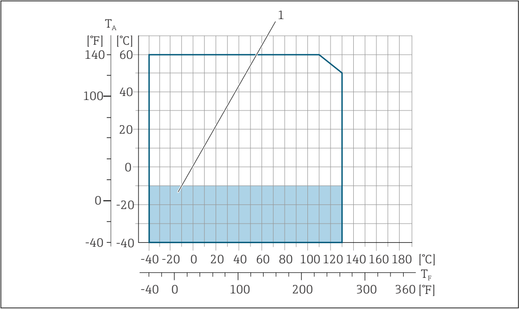
35 PTFE T_A 环境温度 T_F 介质温度 1 彩色区域: -10 ... -40 °C (+14 ... -40 °F)环境温度范围仅适用不锈钢法兰
