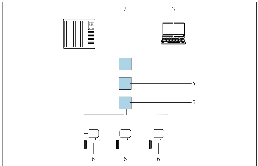
图 67 通过 APL 网络进行远程操作
