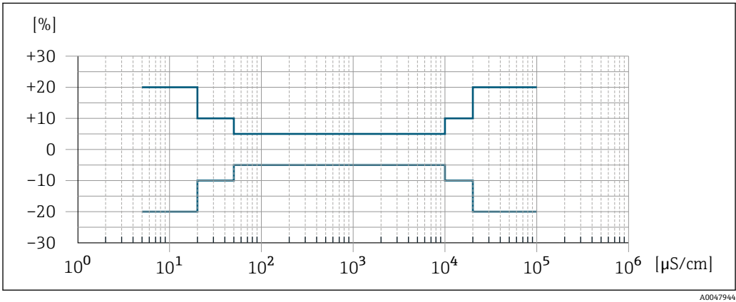
图 26 测量误差 (可选: 订购选项“电导率测量标定”，选型代号 CW)
