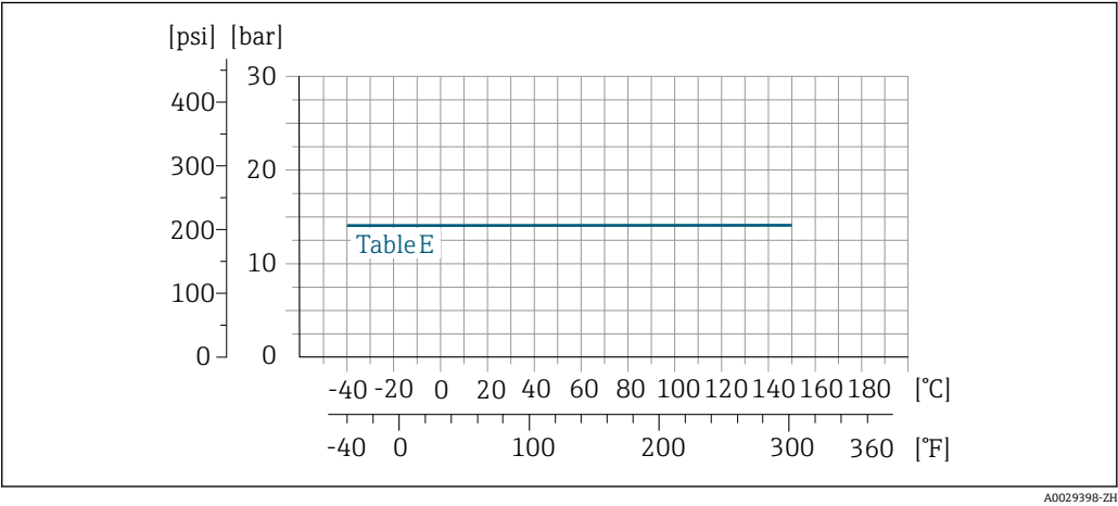
图 41 过程连接材质: 碳钢 A105/S235JRG2/S275JR
