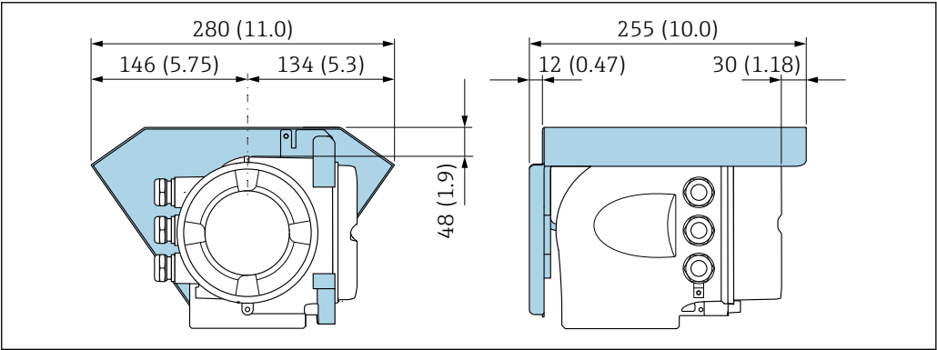
44 Proline 500（模拟）变送器的防护罩的外形尺寸图；单位：mm (in)
