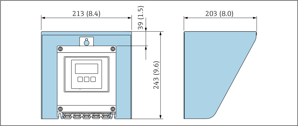
43 Proline 500（数字）变送器的防护罩的外形尺寸图；单位：mm (in)
