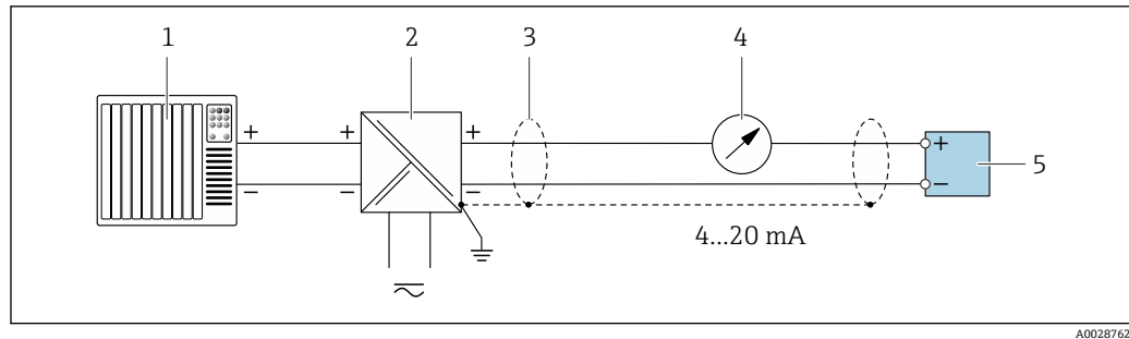
图 3 接线实例：4...20 mA HART 电流输出（无源信号）
