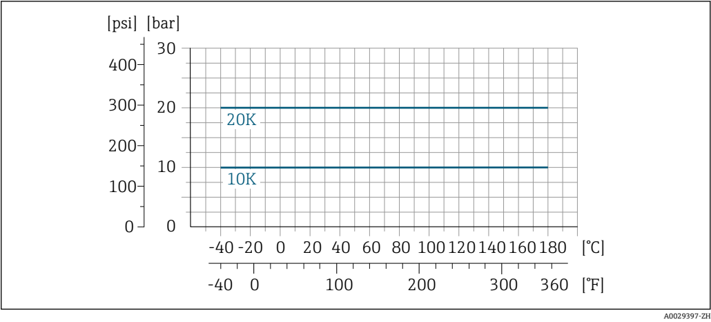
图 40 过程连接材质: 不锈钢 F316L、碳钢 S235JRG2/HII
