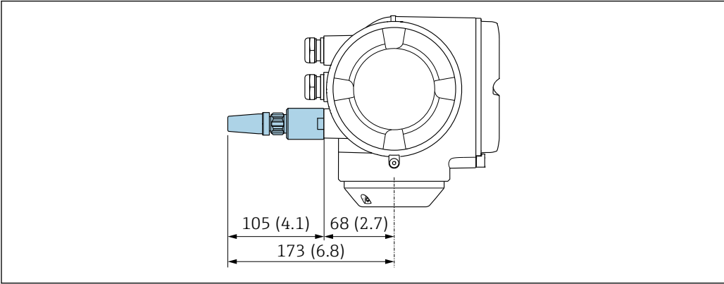
图 53 单位: mm (in)
