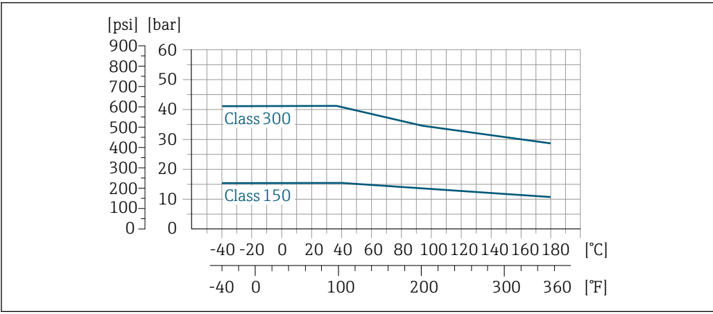
39 过程连接材质：不锈钢 F316L
