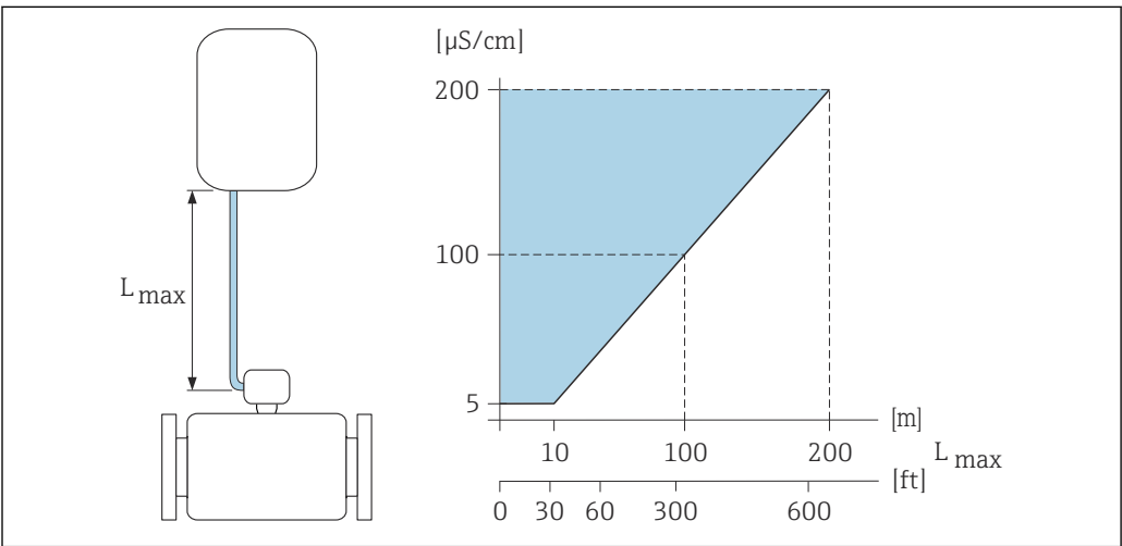
图 27 允许连接电缆长度
