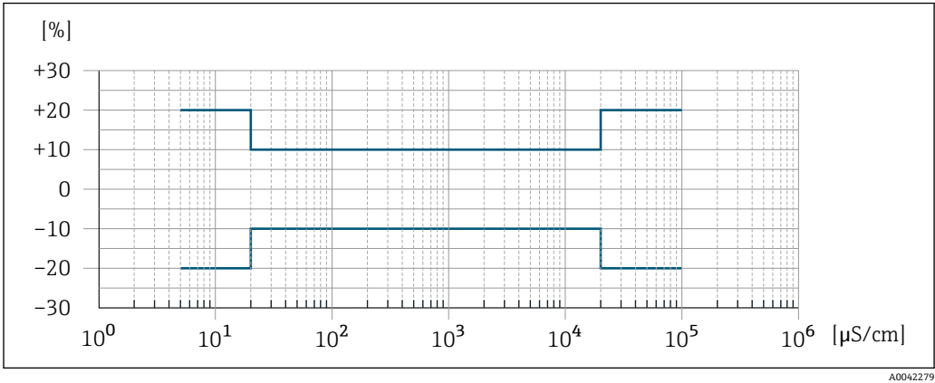
图 25 测量误差 (标准)
