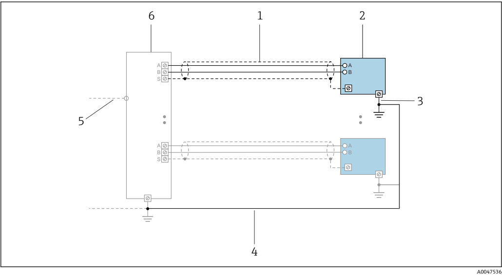
9 接线实例：PROFINET + Ethernet-APL
