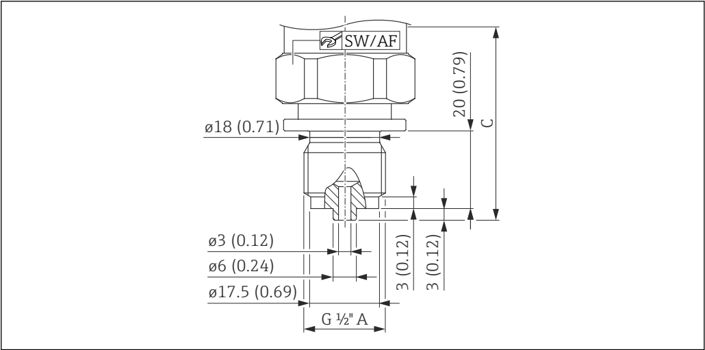
5 Резьба ISO 228 G 1/2" A, EN 837. Единица измерения мм (дюйм)
