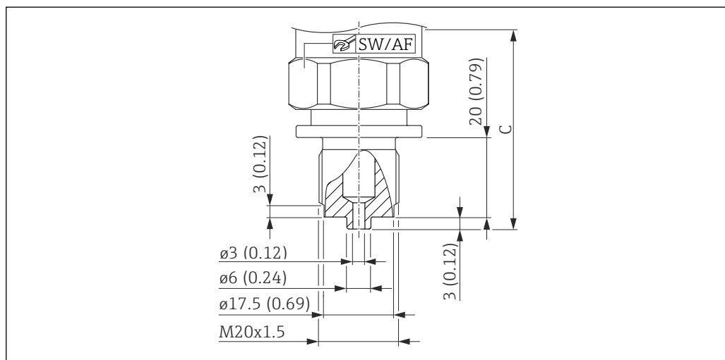
10 DIN 13 M20 x 1,5, EN 837, отверстие 3 мм (0,12 дюйм). Единица измерения мм (дюйм)
