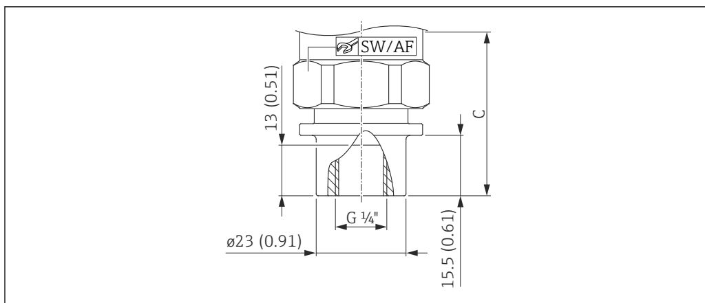
4 Резьба ISO 228 G 1/4" (внутренняя). Единица измерения мм (дюйм)
