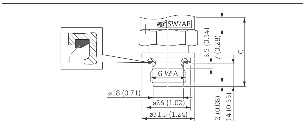
12 DIN 3852, форма E. Диаметр технологической мембраны: 17,2 мм (0,68 дюйм). Единица измерения мм (дюйм)
