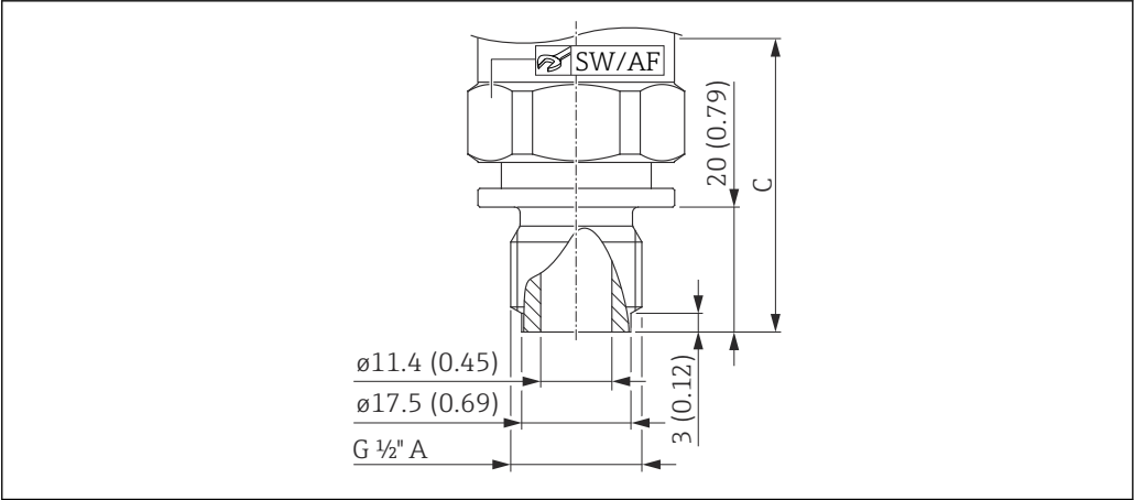
6 Резьба ISO 228 G 1/2" A, отверстие 11,4 мм (0,45 дюйм). Единица измерения мм (дюйм)
