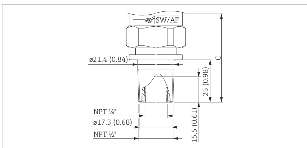
8 ASME 1/2" MNPT, 1/4" FNPT (внутренняя). Единица измерения мм (дюйм)
