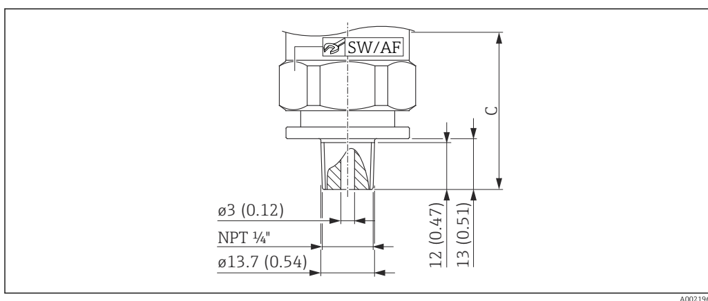
7 ASME 1/4" MNPT, отверстие 3 мм (0,12 дюйм). Единица измерения мм (дюйм)
