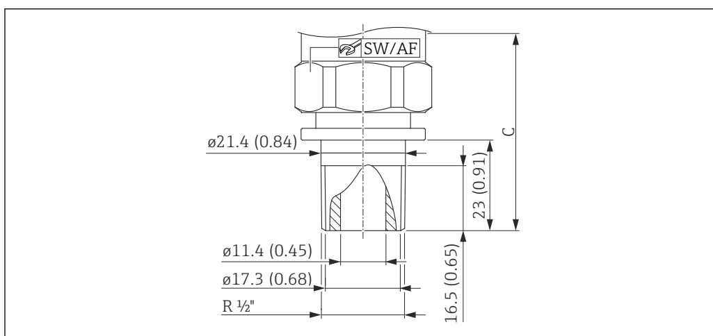
11 Диаметр технологической мембраны: 17,2 мм (0,68 дюйм). Единица измерения мм (дюйм)
