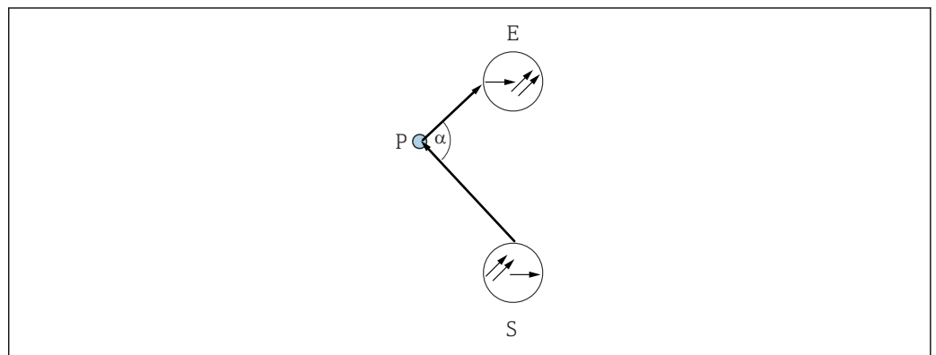
6 90° strooilichtmethode
