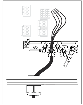
26 Druk de kabel in de aardklem
