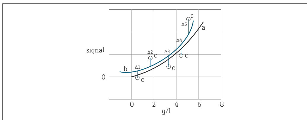
32 Vijfpuntskalibratie
