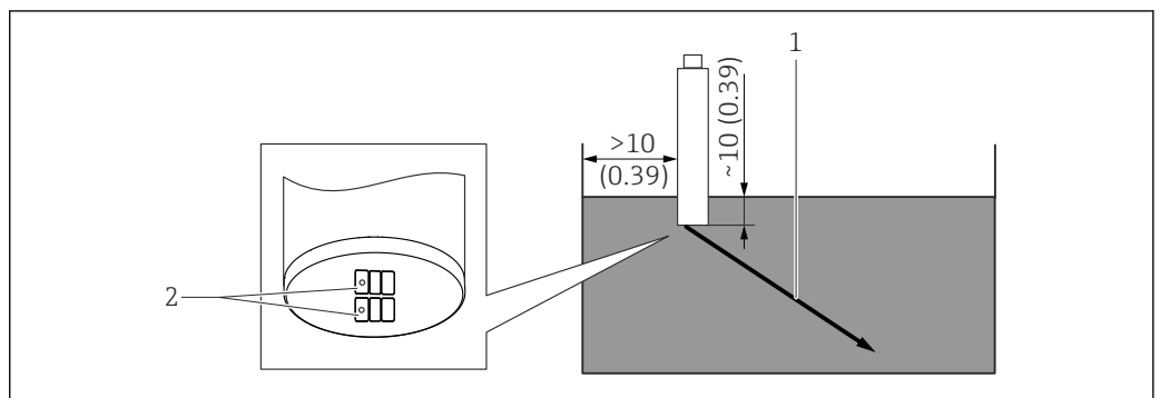
34 Positioneren van de sensor. Afmetingen: mm (in)
