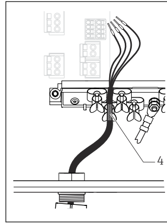
25 Sluit de kabel aan op de aardklem
