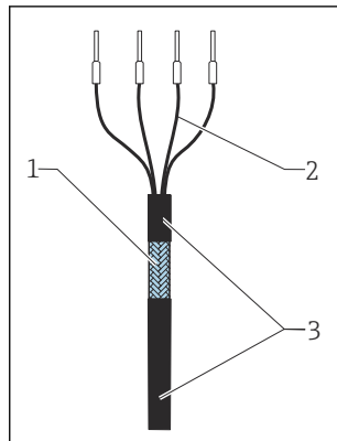
24 Afgesloten kabel
