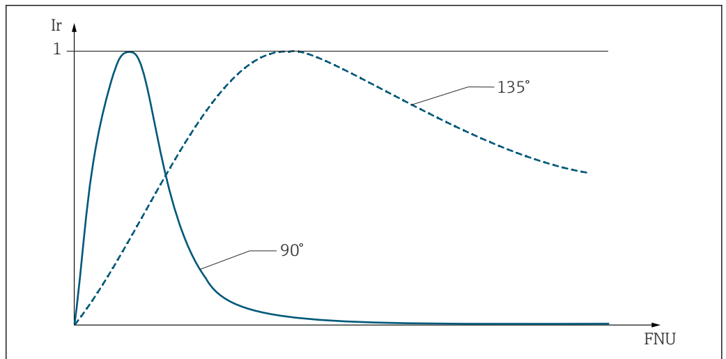
3 Signaalverdeling als functie van de deeltjesdichtheid
