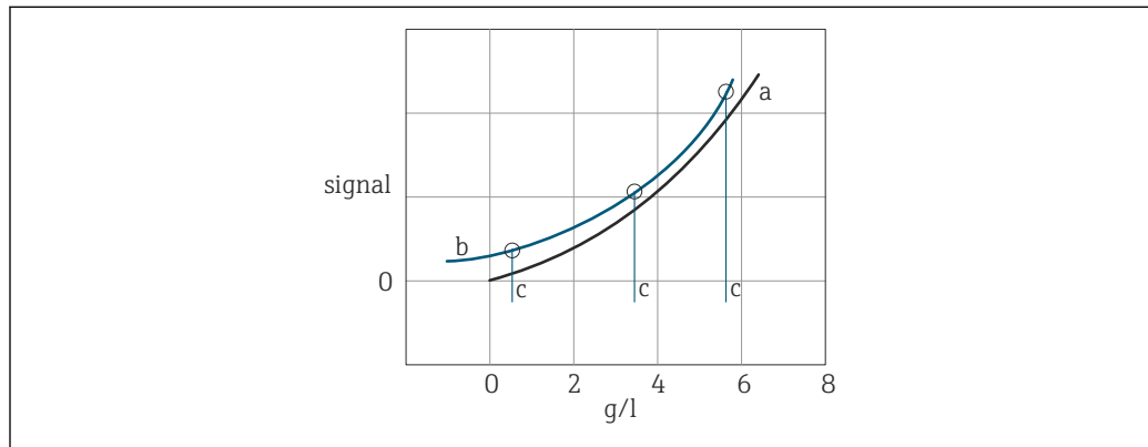
31 Driepuntskalibratie
