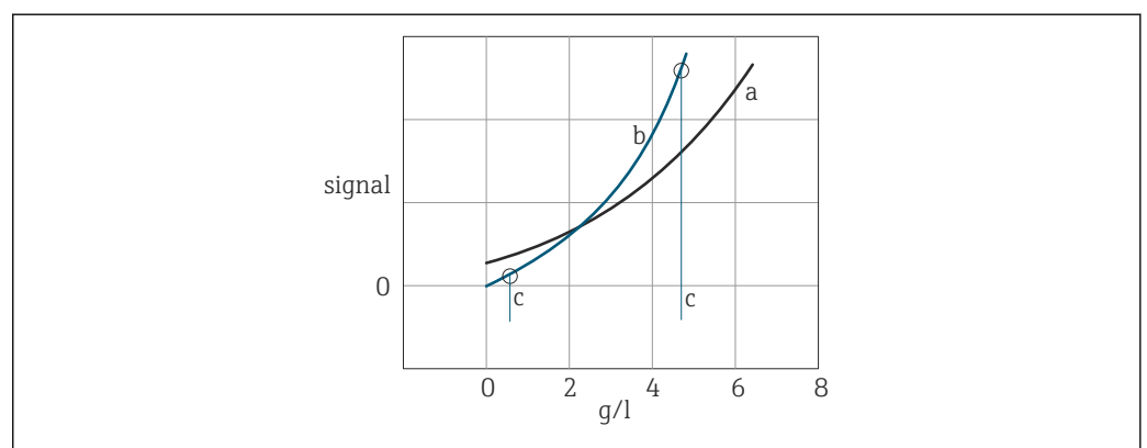
30 Tweepuntskalibratie
