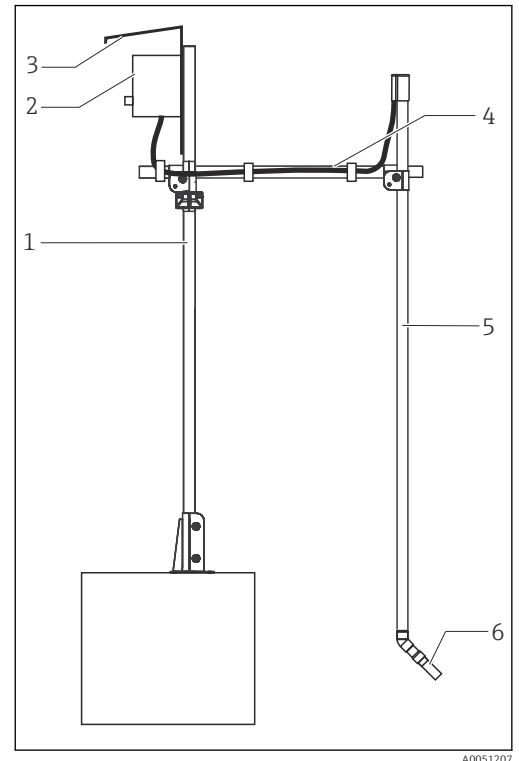
17 Installasjon med stående stolpe
