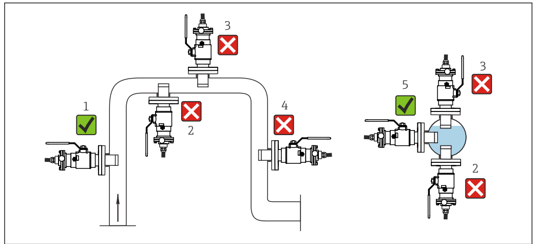
15 Orienteringer og posisjoner (med fellbar enhet CUA451)
