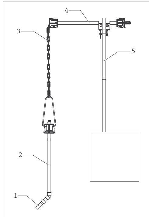
18 Kjettingholder på rekkverk
