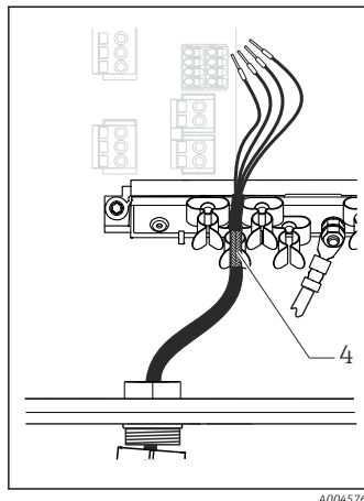
25 Koble kabelen til jordingsklemmen
