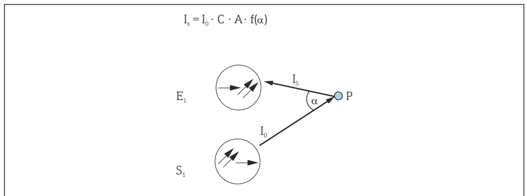
7 Prinsipp for metode for tilbakestrålt lys
