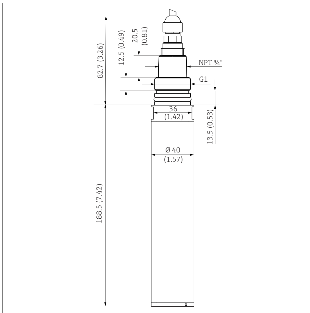
8 Mål. Teknisk enhet: mm (in)
