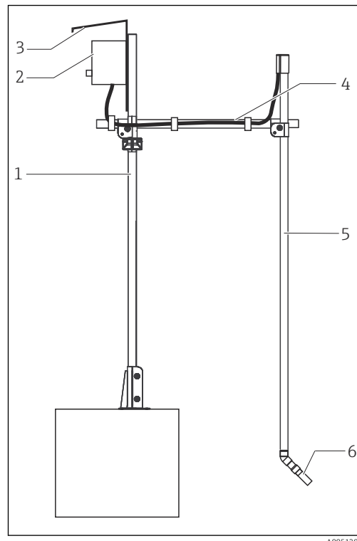
17 Instalare cu stâlp vertical
