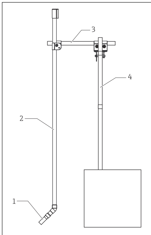
16 Instalarea pe șine
