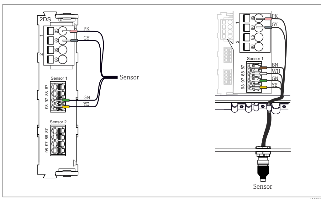
23 Conexiune senzor la intrarea senzorului (stânga) sau prin fișa M12 (dreapta)
