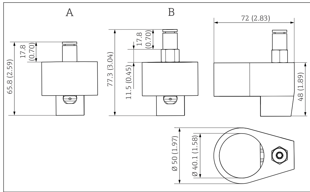
9 Curățare cu aer comprimat. Unitate tehnologică: mm (in)
