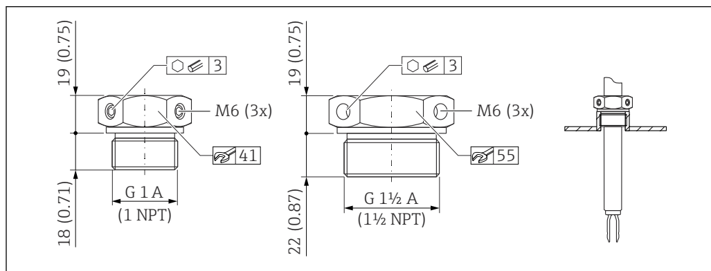
48 Manicotti scorrevoli per il funzionamento non pressurizzato p_e = 0 bar (0 psi). Unità di misura mm (in)
