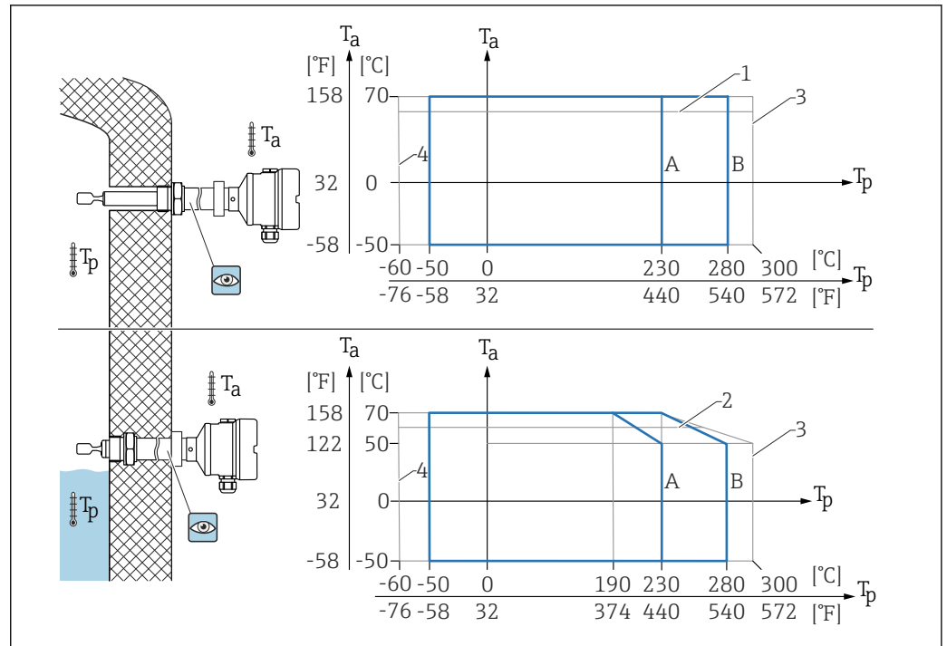
50 Temperatura ambiente ammissibile T_a nella custodia in funzione della temperatura di processo T_p nel silo
