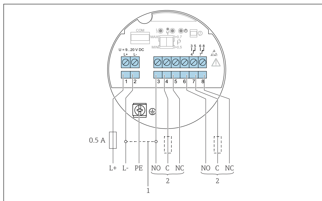
23 Collegamento c.c. con uscita a relè, inserto elettronico FEL64 DC
