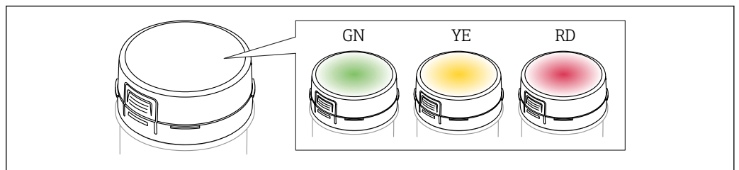
47 Modulo LED, il LED si accende di luce verde (GN), gialla (YE) o rossa (RD)
