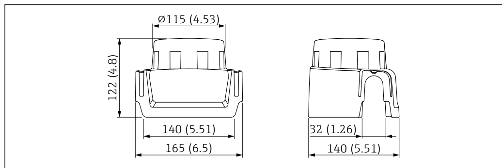
45 Coperchio di protezione per custodia a vano unico, alluminio o 316L. Unità di misura mm (in)
