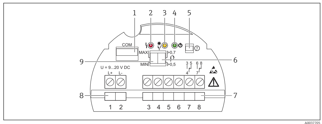
32 Esempio di inserto elettronico FEL64DC
