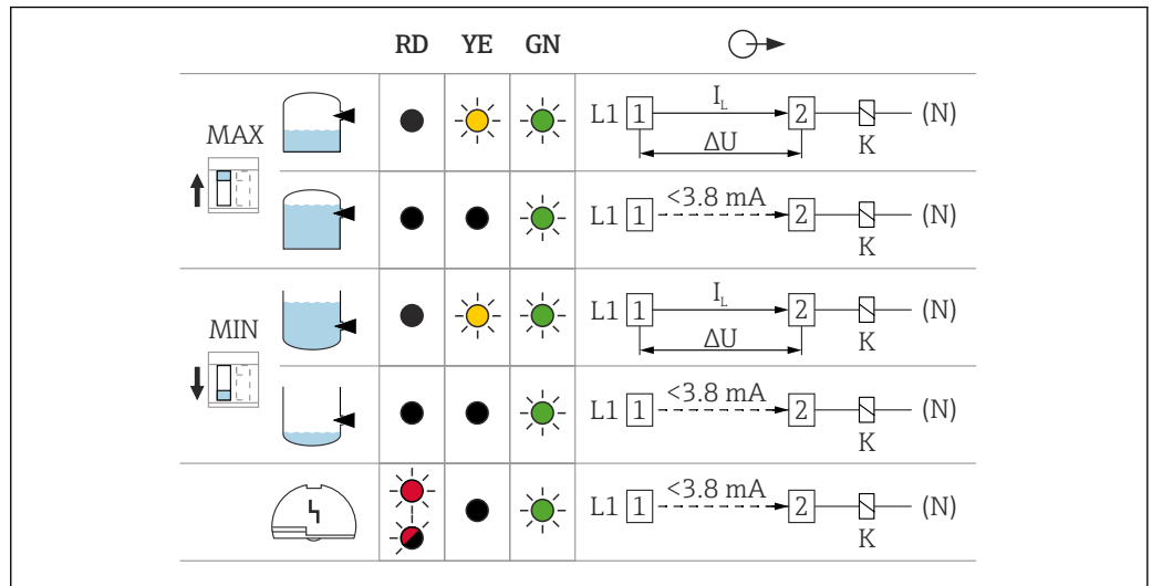
17 Azione dell'uscita di commutazione e segnalazione, inserto elettronico FEL61
