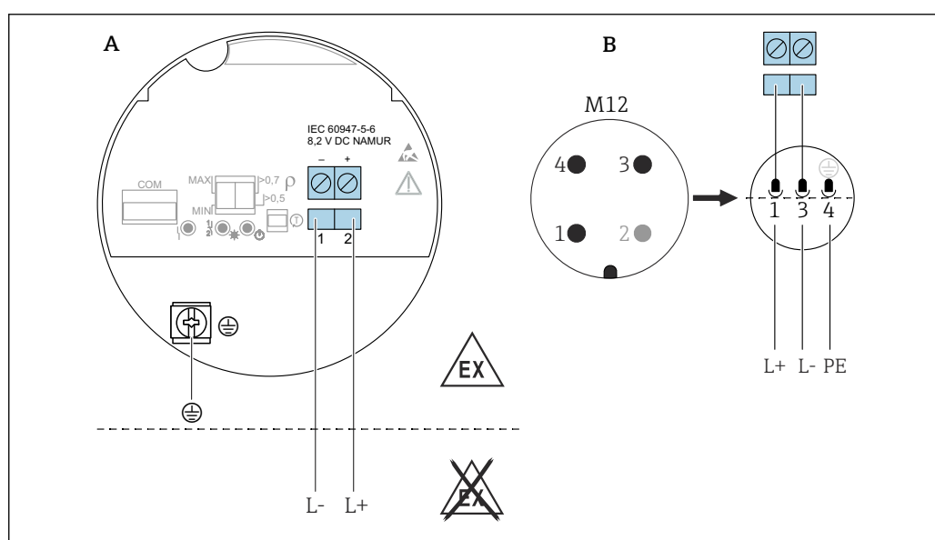
27 NAMUR a due fili \geq 2,2 mA / \leq 1,0 mA, inserto elettronico FEL68
