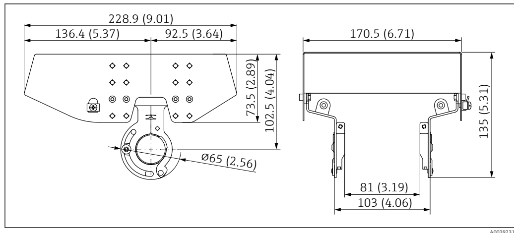
44 Coperchio di protezione per custodia a doppio vano in alluminio. Unità di misura mm (in)
