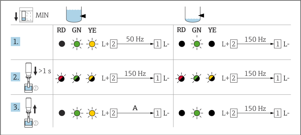
39 Comportamento di commutazione di MIN e segnalazione con FEL67
