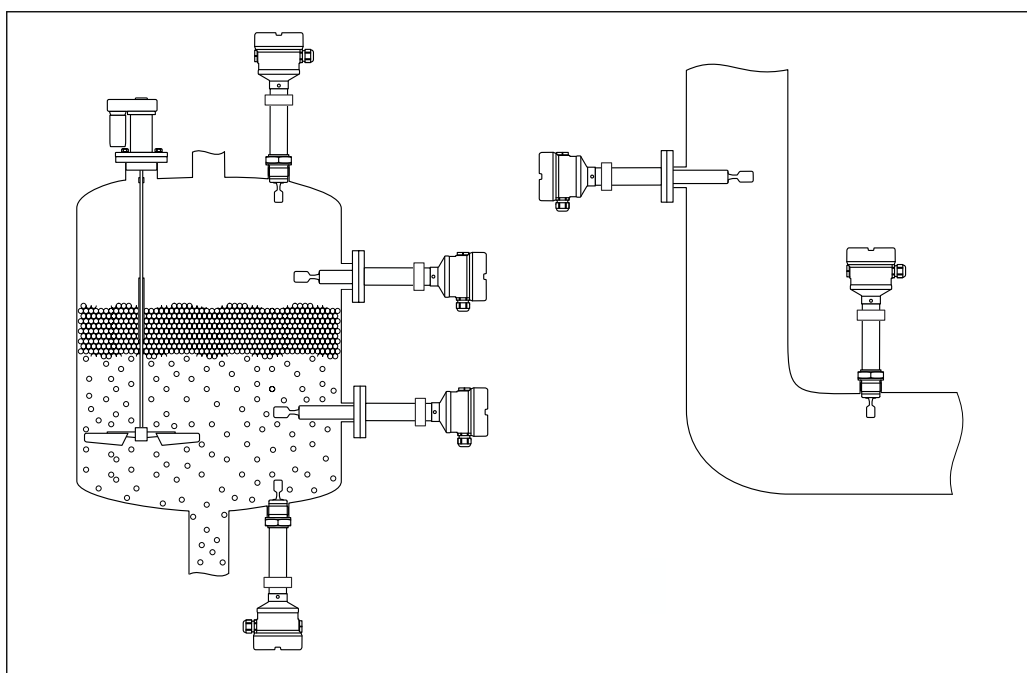
3 Esempi di installazione in silo, serbatoio o tubo
