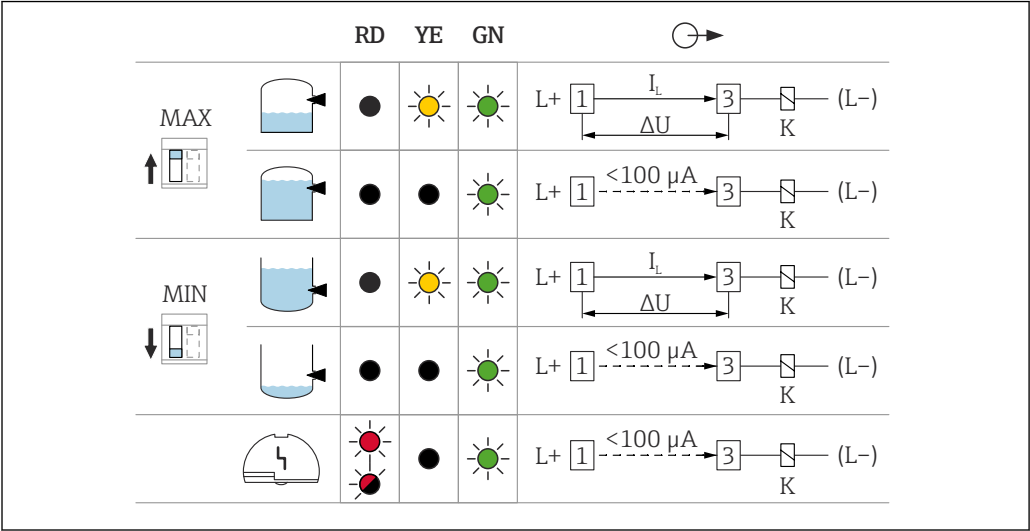
20 Azione dell'uscita di commutazione e segnalazione, inserto elettronico FEL62
