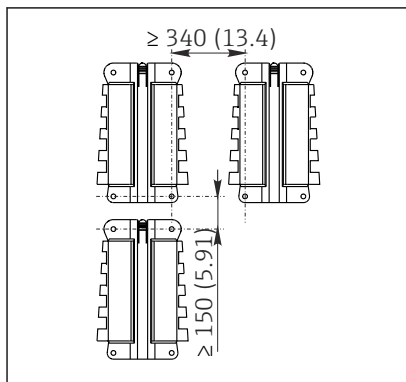
9 Asennusetäisyys mm (tuumaa)
