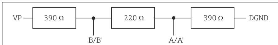
56 Sisäisen väyläpääteen rakenne
