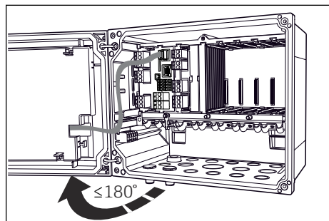
14 Näytön kannen avaaminen, maks. avauskulma 180° (riippuu asennuspaikasta)
