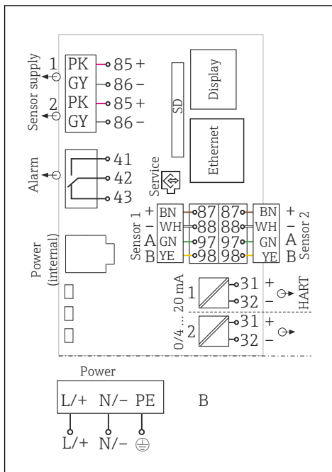
23 Koko kytkentäkaavio käyttäen esimerkkinä BASE2-E:tä ja laajennettua virtalähdettä (B)
