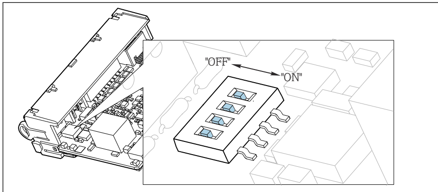
55 Sisäisen väyläpääteen DIP-kytkin
