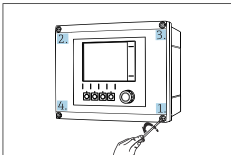
13 Löysää kotelon ruuveja ristiin Phillips-ristipääruuvimeisselillä
