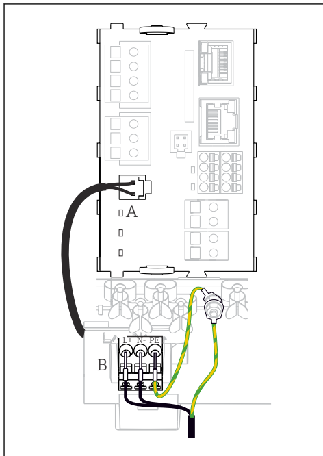
22 Virtalähteen kytkentä käyttäen esimerkiksi BASE2-E:tä
