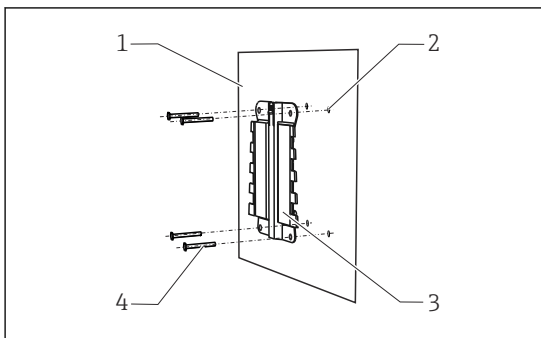
10 Seinäasennus
