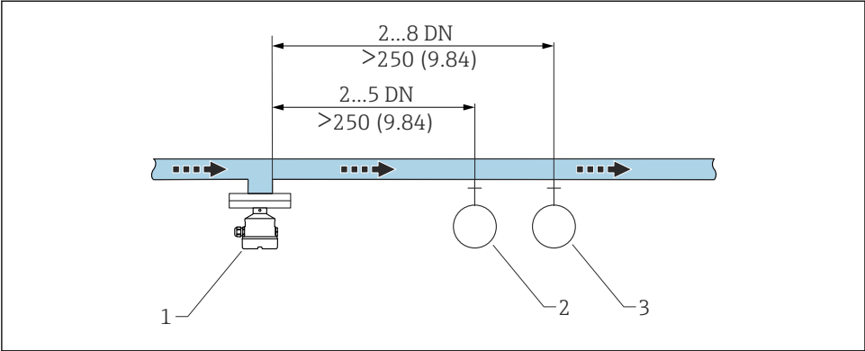
6 Монтаж прямого участка после прибора. Единица измерения мм (дюйм)
