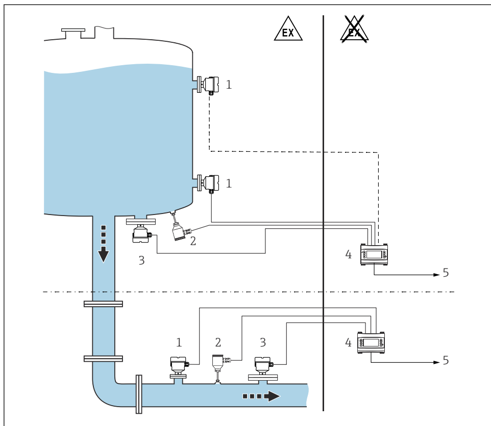
16 Измерение плотности в сочетании с электронным преобразователем Density Computer FML621
