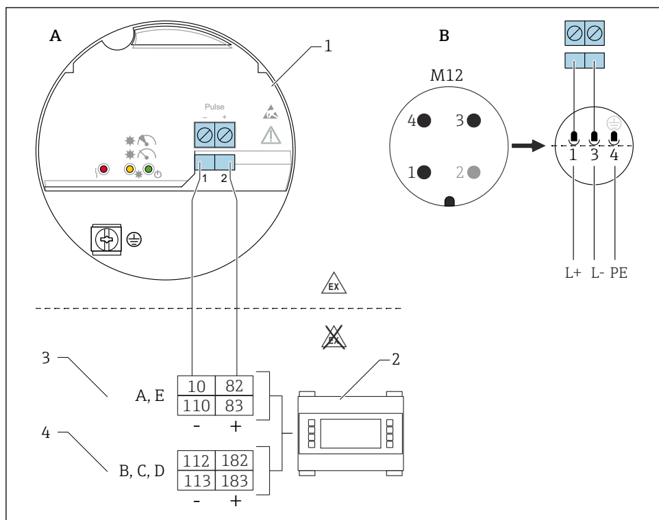
15 Схема подключения: соединение электронной вставки FEL60D с электронным преобразователем FML621
