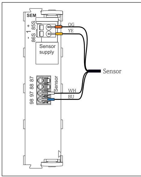
33 Spektrometertilkobling til SEM/modul
