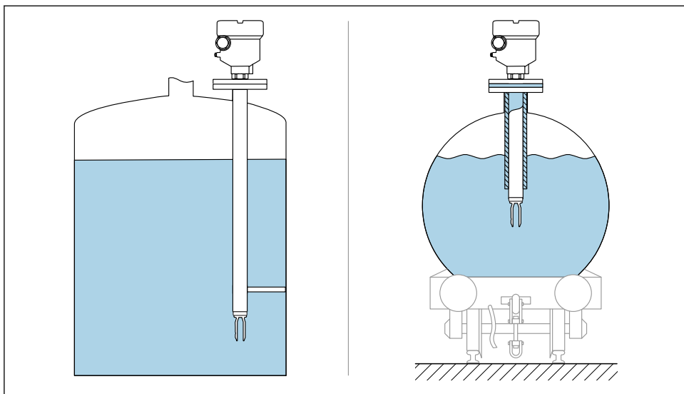
7 Podepření pro případ dynamického zatížení
