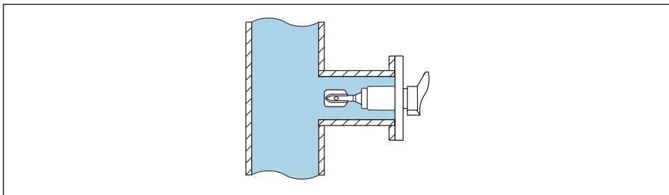
3 Příklad instalace v potrubí mimo přímý tok média
