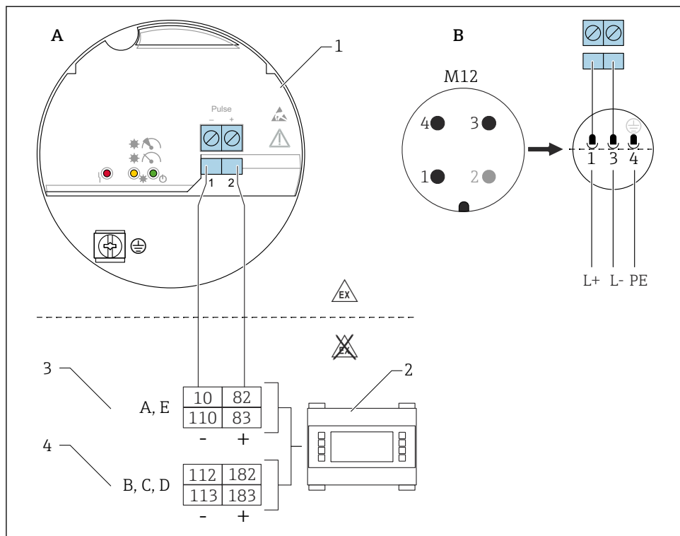
12 Schéma připojení: elektronická vložka FEL60D připojení k přepočítávači hustoty FML621
