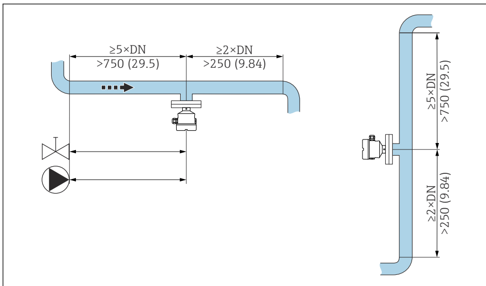
4 Instalace náběžné délky potrubí. Jednotka měření mm (in)
