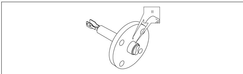
8 Poloha vibrační vidličky při vodorovné instalaci v nádobě pomocí označení
