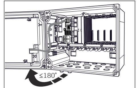
24 Открывание крышки дисплея (не более чем на 180°, зависит от монтажного положения)
