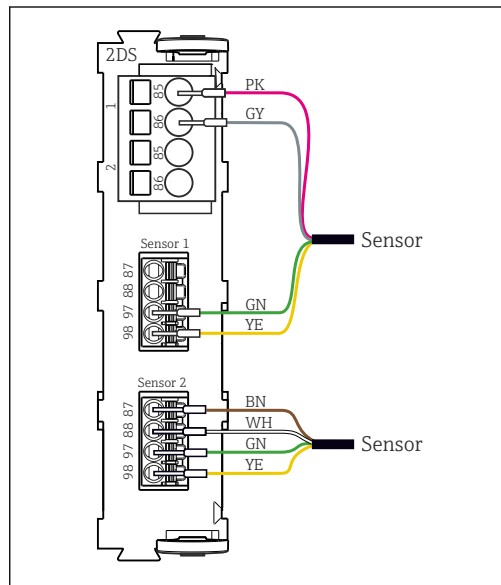
37 Датчики с дополнительным источником питания и без него на модуле датчика 2DS
