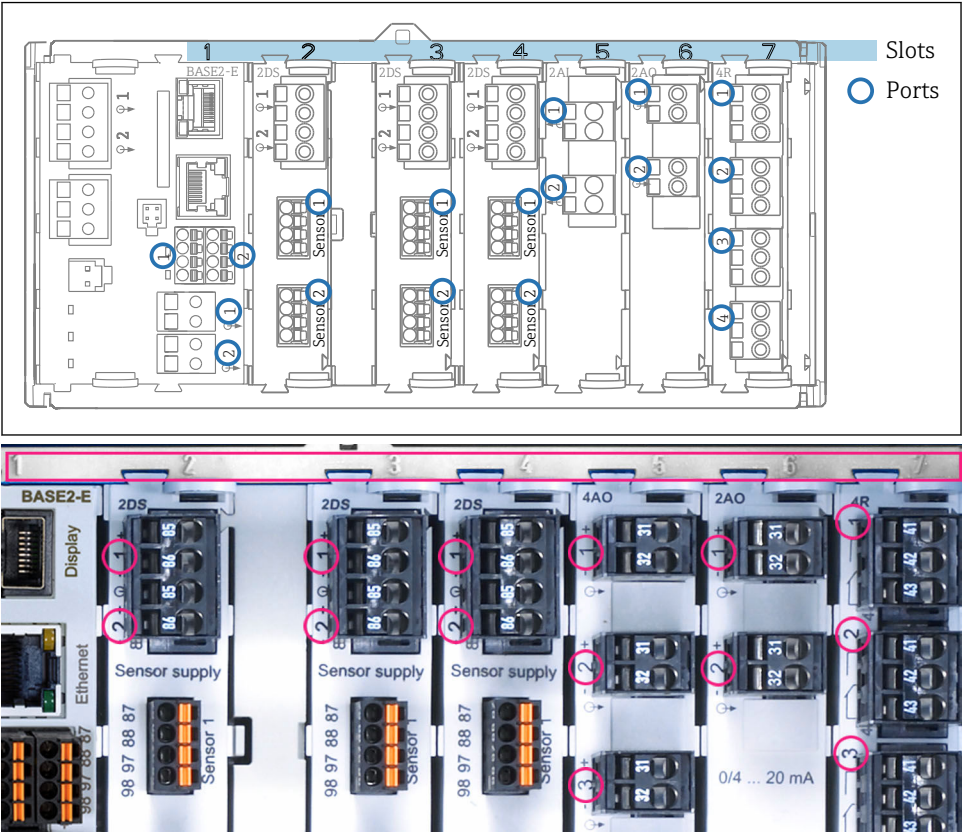
4 Назначение гнезд и портов аппаратных модулей
