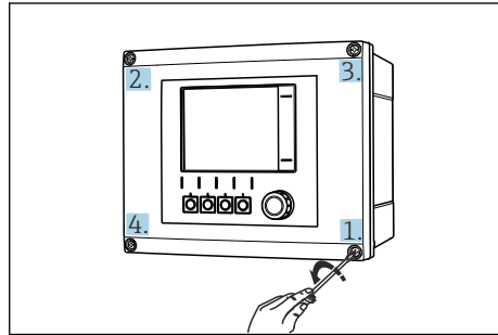
23 Ослабьте винты корпуса в перекрестном порядке отверткой с крестообразным наконечником
