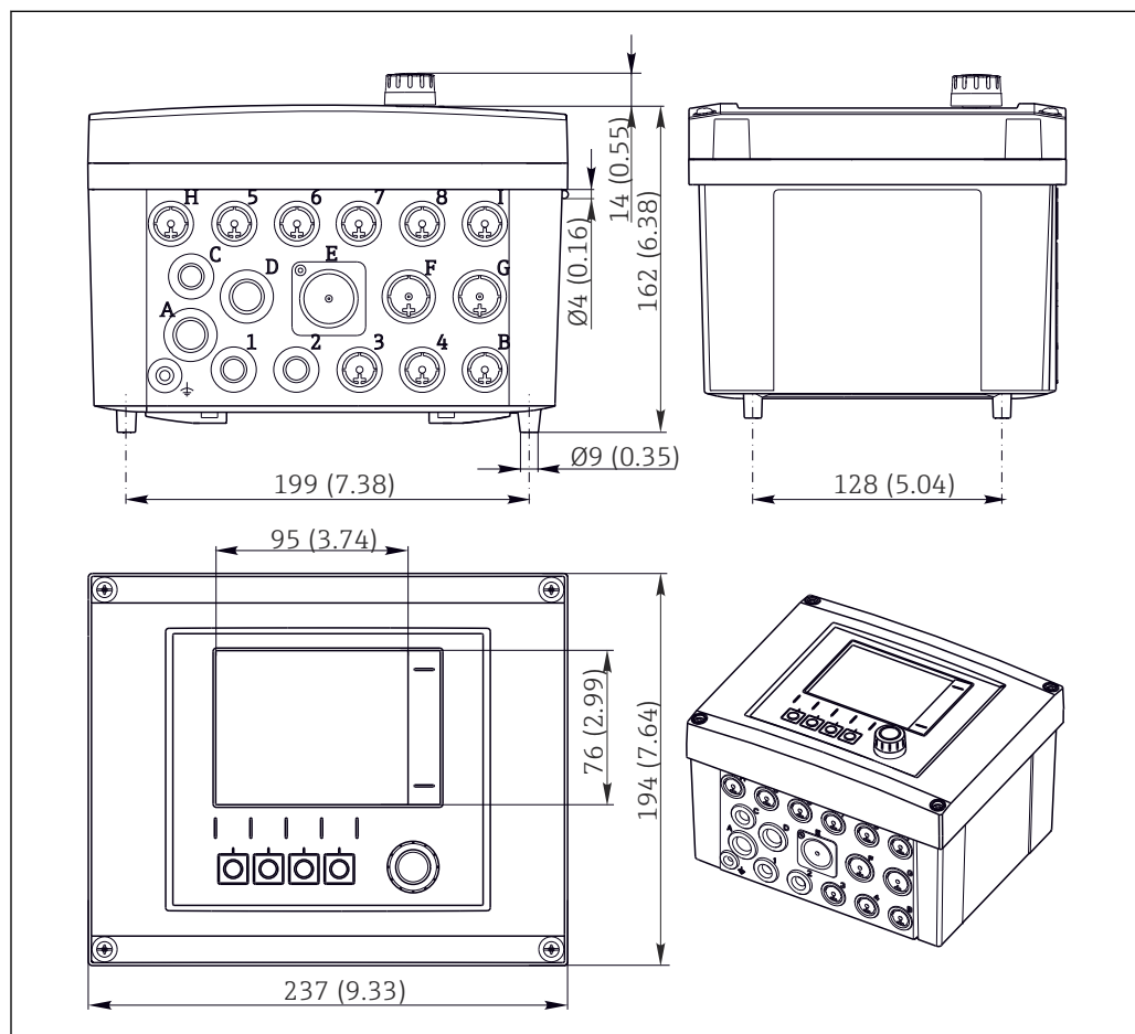
7 Размеры полевого корпуса в мм (дюймах)
