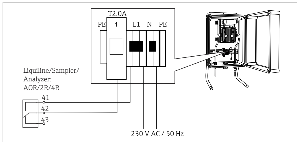
53 Подключение блока очистки для CAS40D
