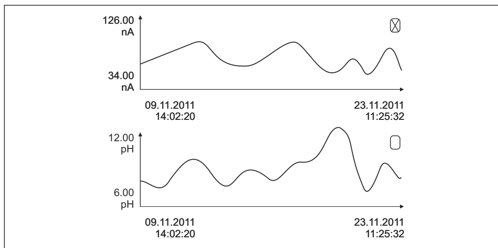
89 Одновременное отображение двух графиков, выбран верхний
