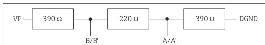
68 Структура внутреннего терминирования
