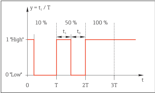
76 Типичное применение: электромагнитный клапан
