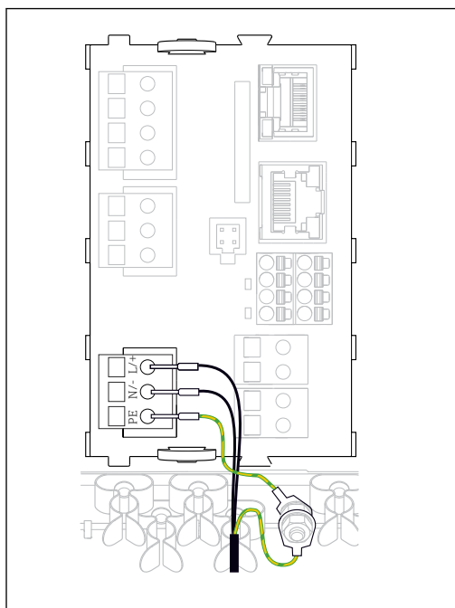
29 Подключение электропитания на примере модуля BASE2-H или -L
