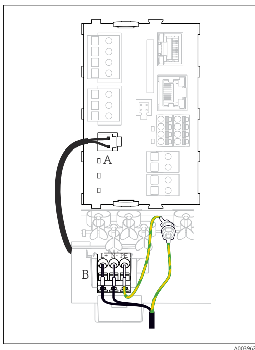
32 Подключение электропитания на примере модуля BASE2-E
