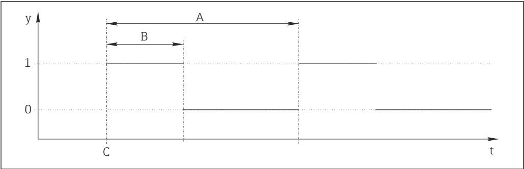
84 Схема сигнала реле времени t Временная шкала y Уровень сигнала (1 – вкл., 0 – выкл.) A Период B Длительность сигнала C Время начала (Дата запуска, Время зап.)
