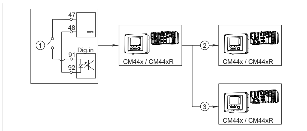
79 Пример для централизованного управления очисткой
