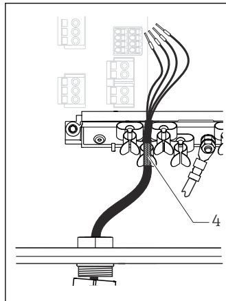
27 Подсоединение кабеля к заземляющему зажиму
