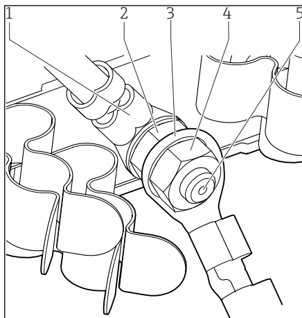
31 Защитное заземление или соединение с землей
