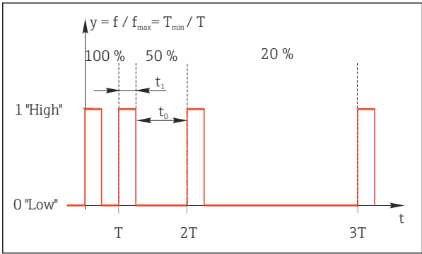
77 Типичное применение: дозировочный насос
