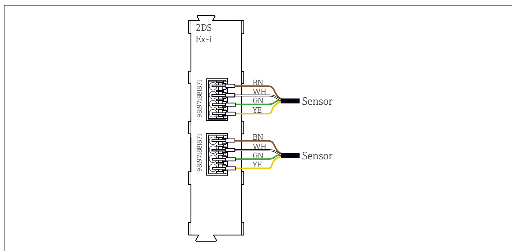
40 Датчики без дополнительного источника питания на коммуникационном модуле датчика 2DS Ex-i
