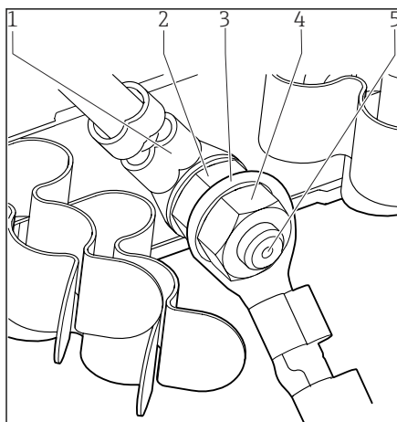
34 Защитное заземление или соединение с землей
