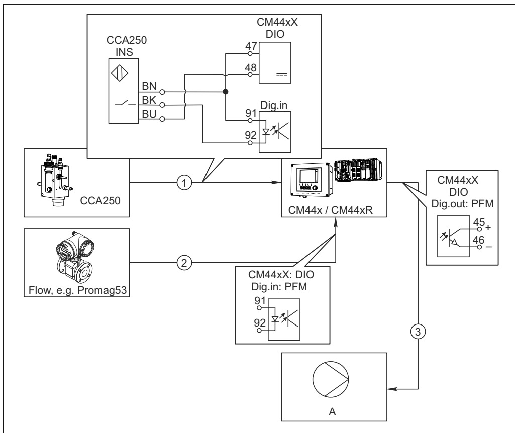
78 Пример контроля над содержанием хлора с прямым управлением
