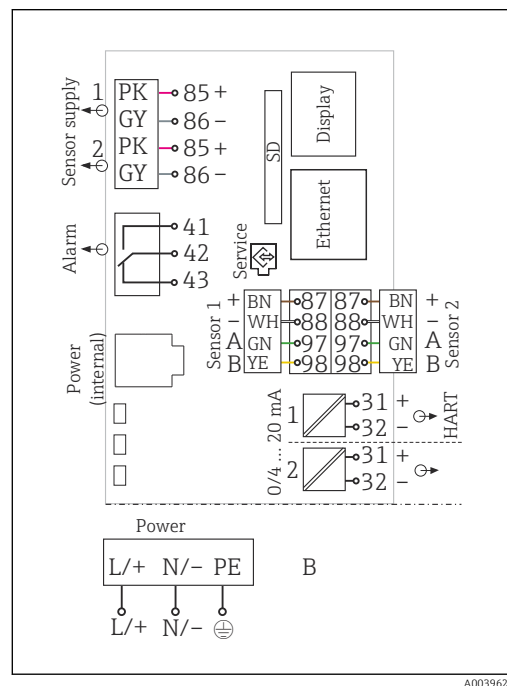
33 Полная электрическая схема на примере модуля BASE2-E и выносного блока питания (B)
