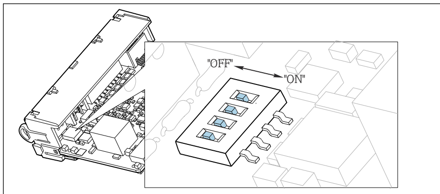
67 DIP-переключатель для внутреннего терминирования
