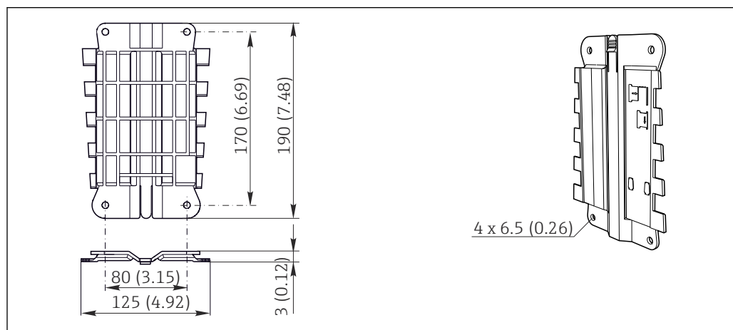
8 Монтажная пластина. Единица измерения: миллиметр (дюйм)
