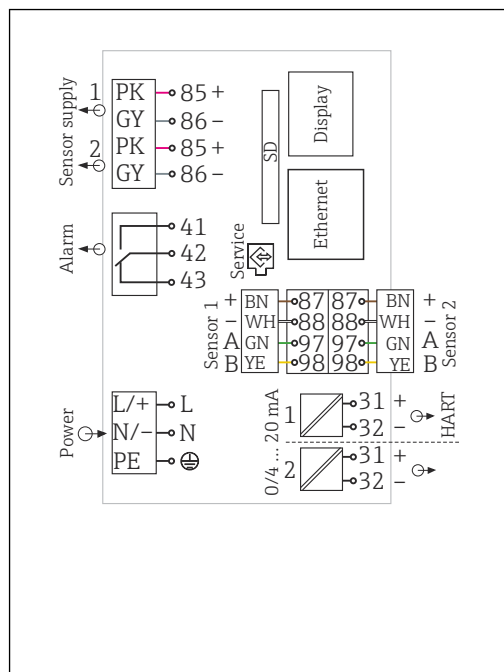
30 Полная электрическая схема на примере модуля BASE2-H или -L
