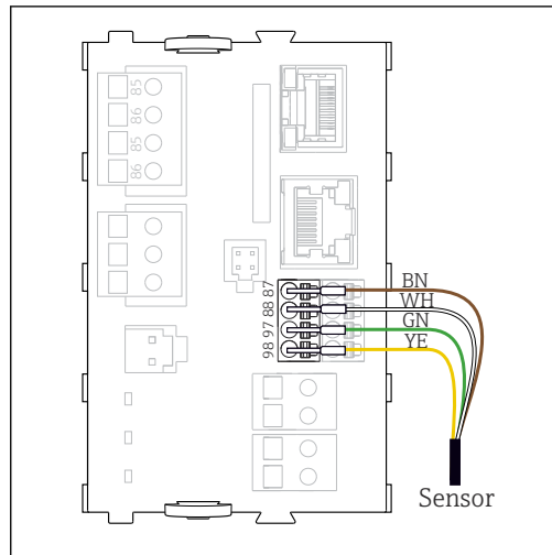
35 без дополнительного электропитания
