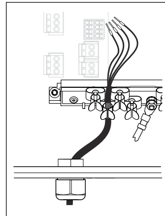
28 Вдавливание кабеля в заземляющий зажим
