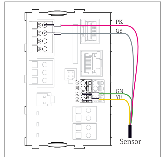
36 с дополнительным электропитанием
