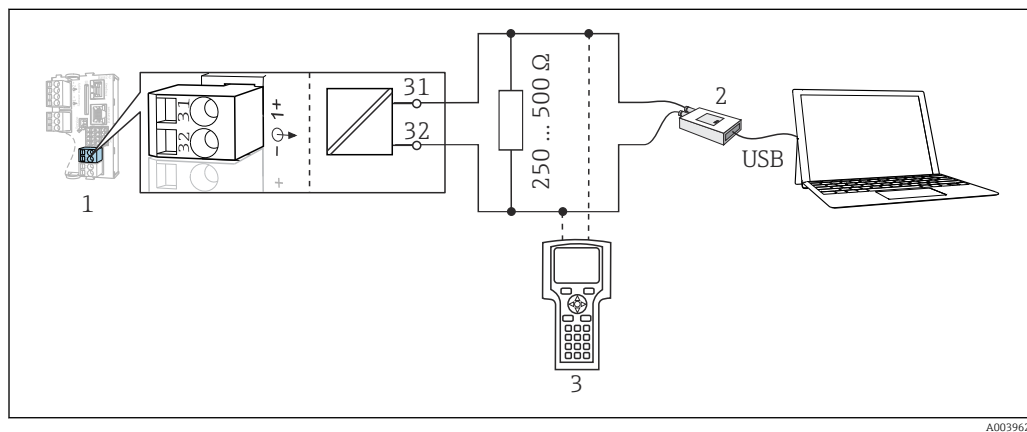
22 Передача данных по протоколу HART посредством модема
