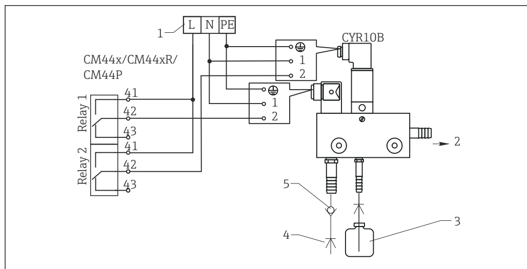
54 Подключение блока очистки инжектора CYR10B
