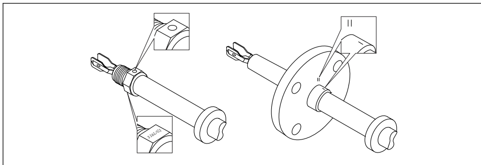
8 Posizione del diapason quando installato orizzontalmente nel silo utilizzando il contrassegno
