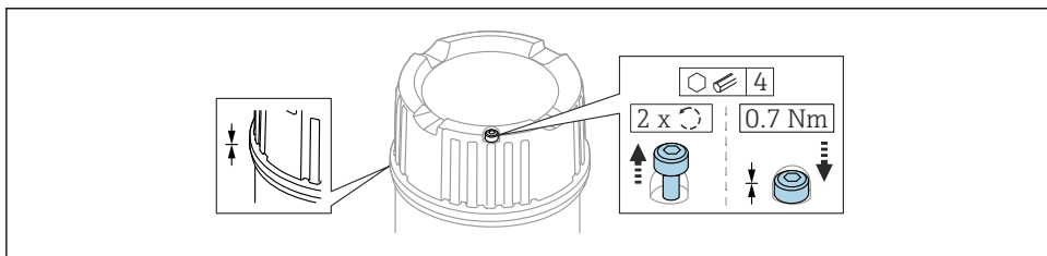
12 Coperchio con vite di fissaggio
