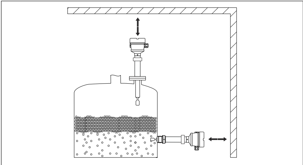
6 Considerazione delle distanze libere al di fuori del serbatoio
