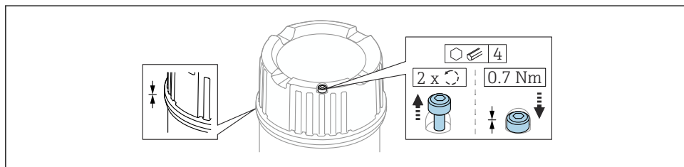
12 Capac cu șurub de fixare
