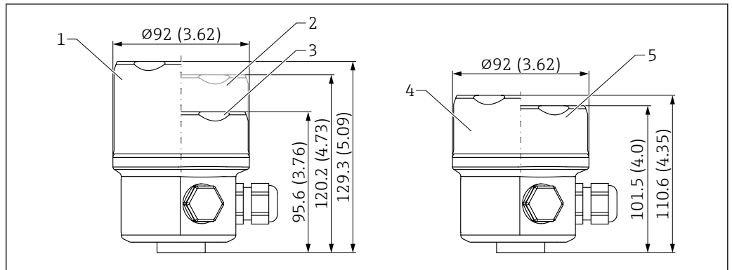
34 Dimensioni della custodia a vano unico, 316L, igienica. Unità di misura mm (in)
