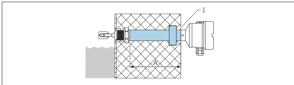
36 Distanziale di temperatura con accoppiatore in vetro a tenuta gas
