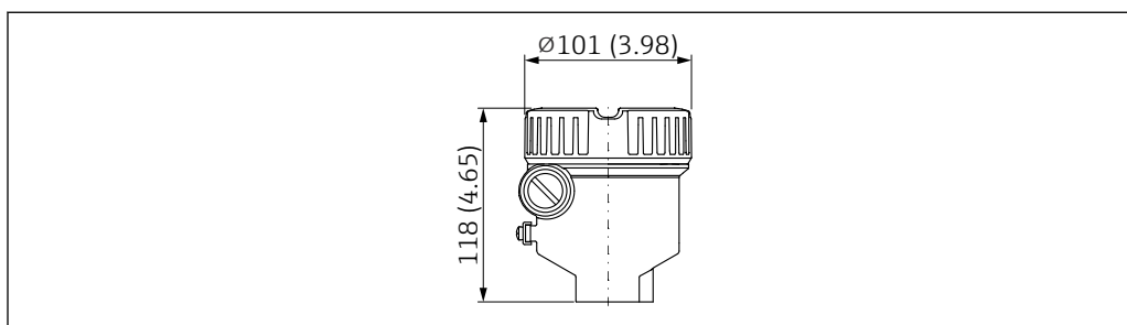
33 Dimensioni della custodia 316L a vano unico; anche con Ex d/XP, a prova di polveri infiammabili; coperchio senza vetro di ispezione. Unità di misura mm (in)
