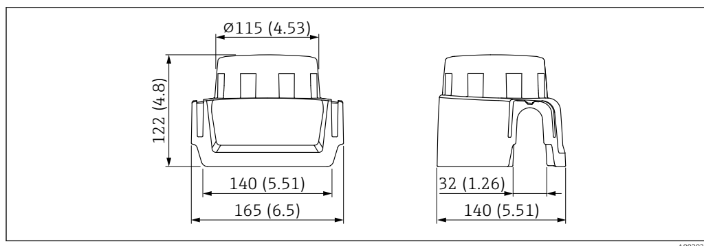
56 Coperchio di protezione per custodia a vano unico, alluminio o 316L. Unità di misura mm (in)
