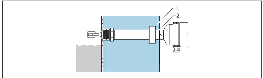
26 Silo coibentato
