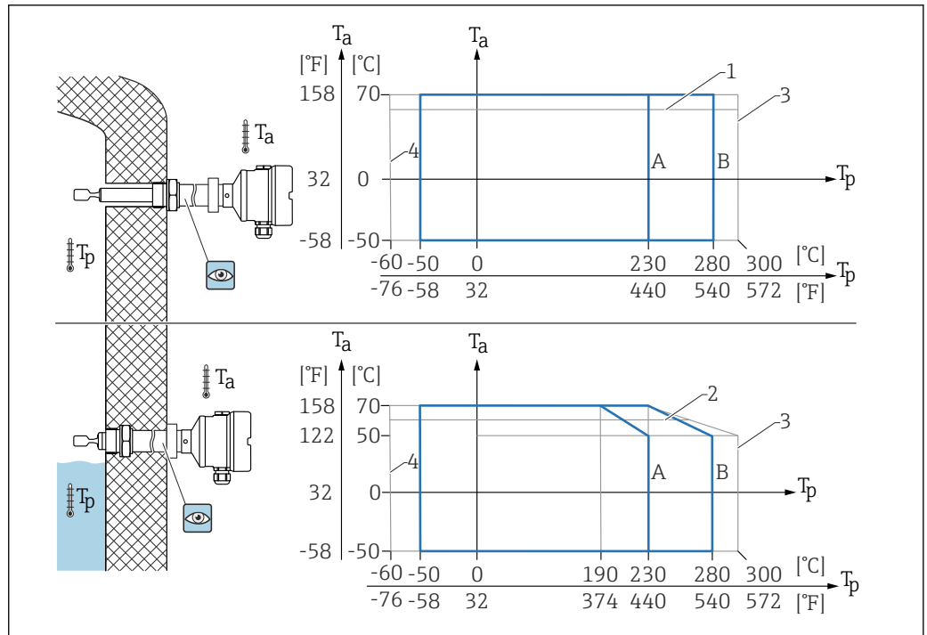
28 Temperatura ambiente ammissibile T_a nella custodia in funzione della temperatura di processo T_p nel silo
