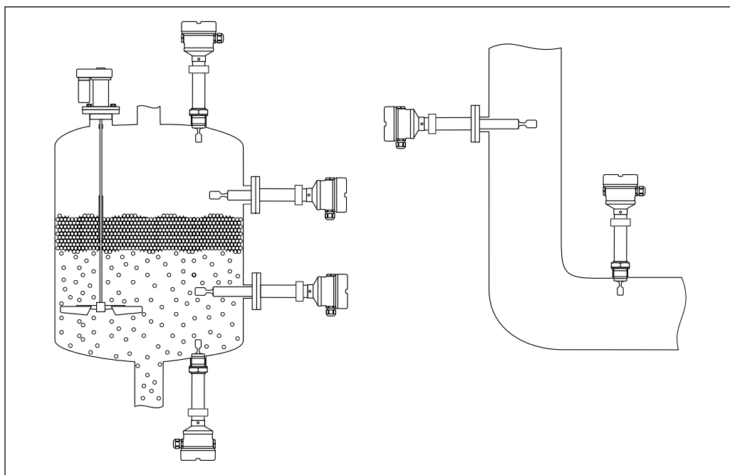
18 Esempi di installazione in silo, serbatoio o tubo
