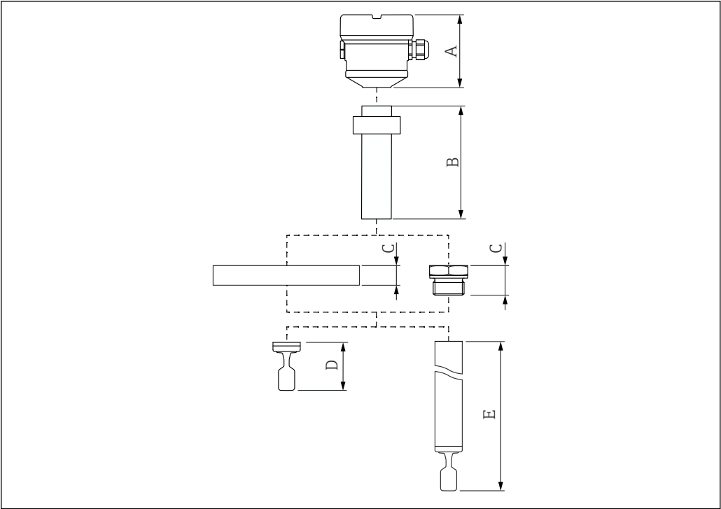
29 Componenti per determinare l'altezza del dispositivo
