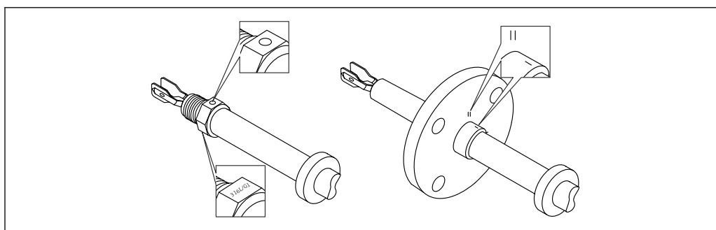
■ 23 Posizione del diapason quando installato orizzontalmente nel silo utilizzando il contrassegno
