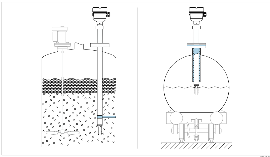
27 Esempi di supporto in caso di carico dinamico
