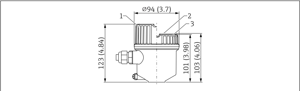
30 Dimensioni della custodia a vano unico, in plastica. Unità di misura mm (in)
