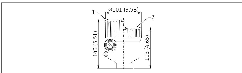
32 Dimensioni della custodia a vano unico, in alluminio, rivestita; con Ex d/XP, a prova di polveri infiammabili. Unità di misura mm (in)
