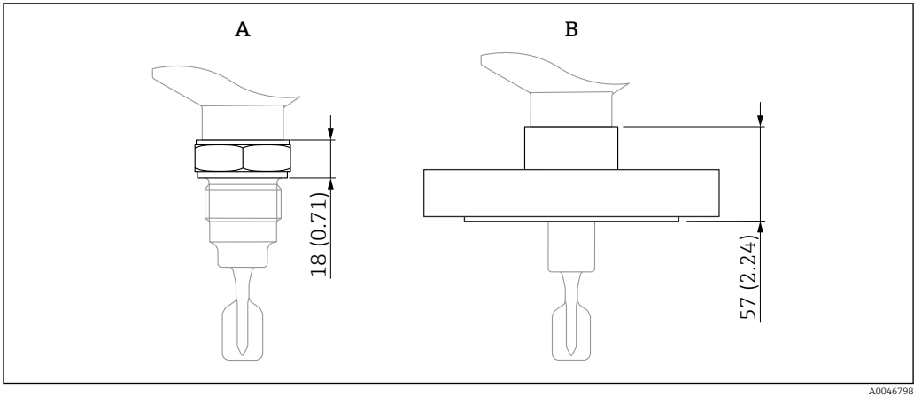
40 Specifiche dell'altezza massima per le connessioni al processo
