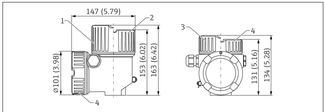
35 Dimensioni della custodia a doppio vano, a L, in alluminio, rivestita; anche con Ex d/XP, a prova di polveri infiammabili. Unità di misura mm (in)
