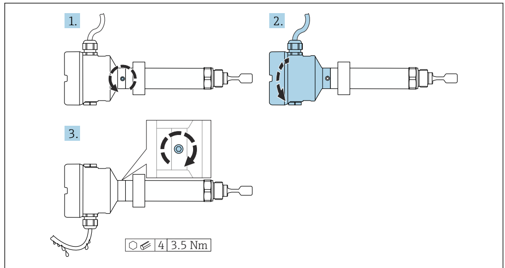
25 Custodia con vite di bloccaggio esterna e anello salvagoccia
