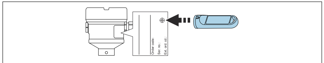
51 Verifica funzionale mediante magnete di prova
