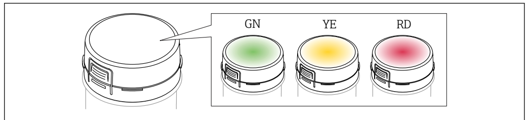
52 Modulo LED: il LED si accende in verde (GN), giallo (YE) o rosso (RD)
