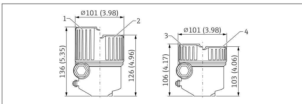
31 Dimensioni della custodia a vano unico, in alluminio, rivestita. Unità di misura mm (in)
