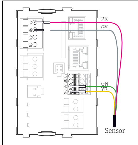
31 Memosens センサ、追加供給電圧あり
