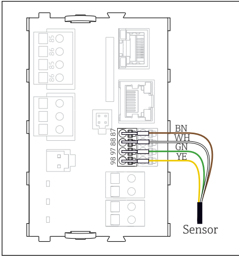
30 Memosens センサ、追加供給電圧なし
