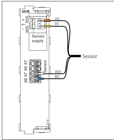
33 スペクトロメータの SEM モジュールへの接続
