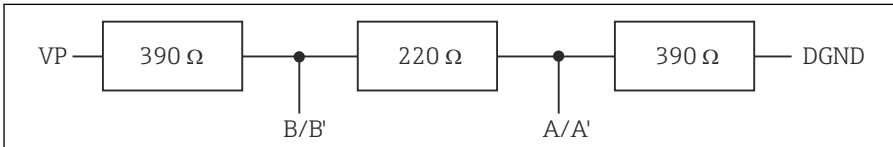
図 62 内部終端の構造
