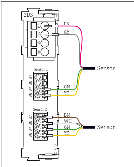
32 センサモジュール 2DS における追加供給電圧付きセンサと追加供給電圧なしのセンサ
