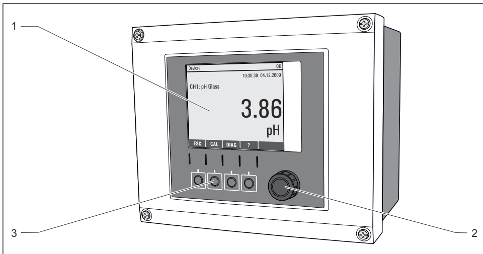
図 66 操作の概要（フィールドハウジングを使用した例）
