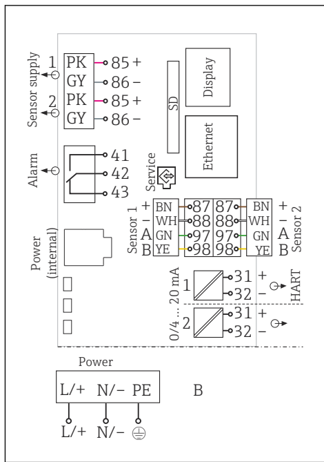
図 27 BASE2-E および外部電源ユニット (B) を使用した全体配線図例
