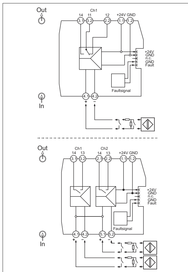
3 Klembezetting van RLN22: 1-kanaals versie (boven), 2-kanaals versie (onder)
