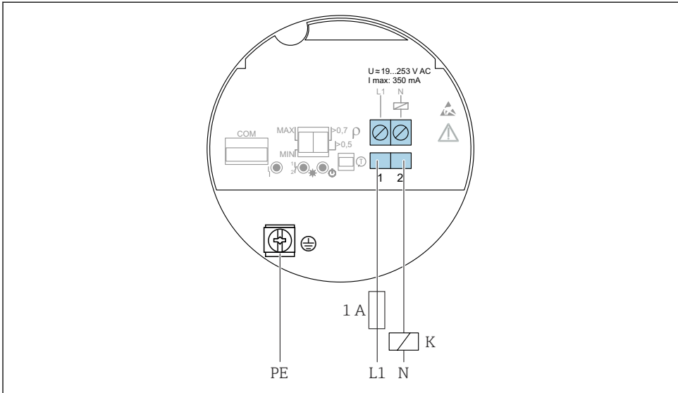
13 2선식 AC, 기판 FEL61
