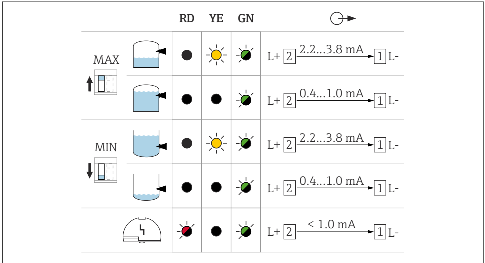
☞ 25 스위치 출력 및 신호 동작, 기판 FEL68
