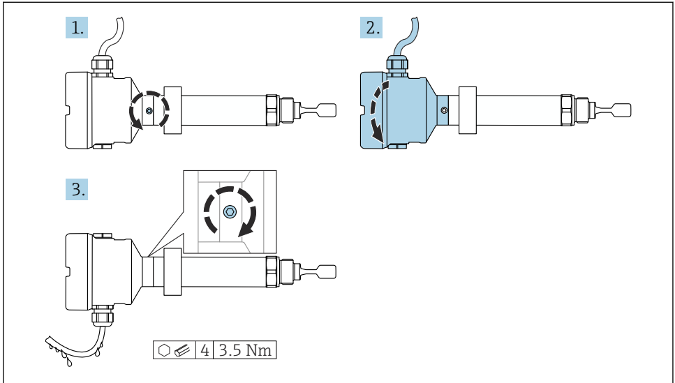
☐ 11 외부 잠금 나사가 있고 케이블을 아래로 늘어뜨린 하우징
