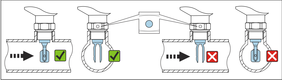
☞ 9 배관에 설치(포크 위치 및 마킹 고려)
