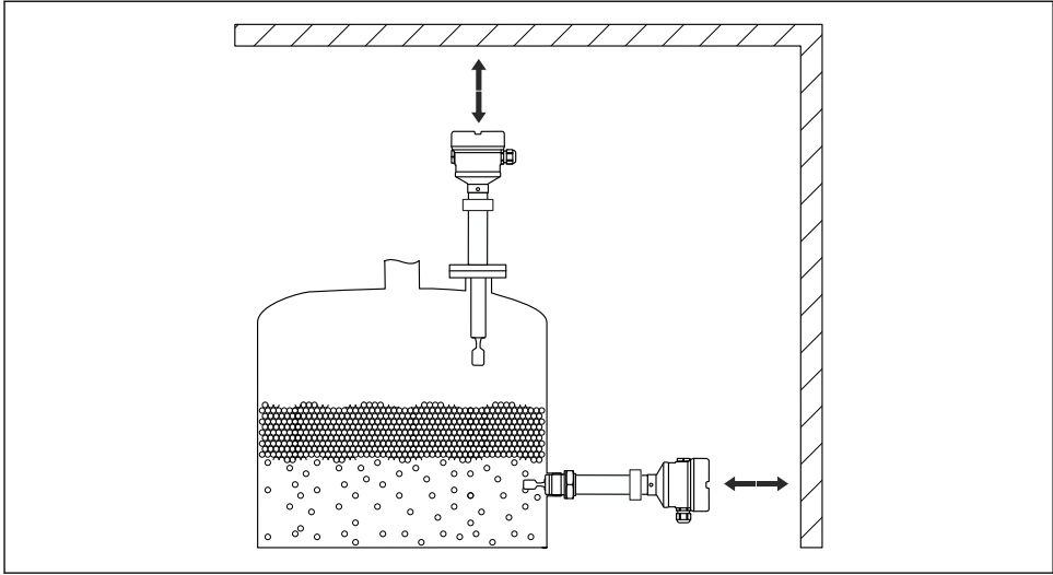
6 탱크 외부의 간격 고려
