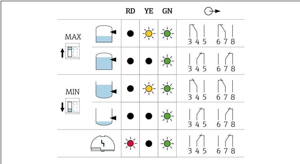
■ 19 스위치 출력 및 신호 동작, 기판 FEL64
