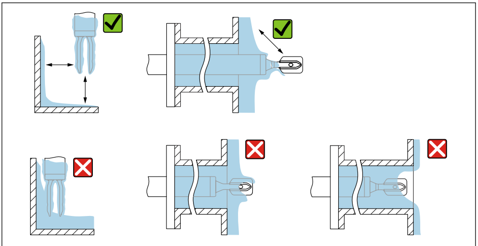
☞ 5 고점성 프로세스 유체용 설치 예
