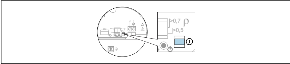
29 기판 FEL61/62/64/64DC/67/68의 기능 테스트 키 위치
