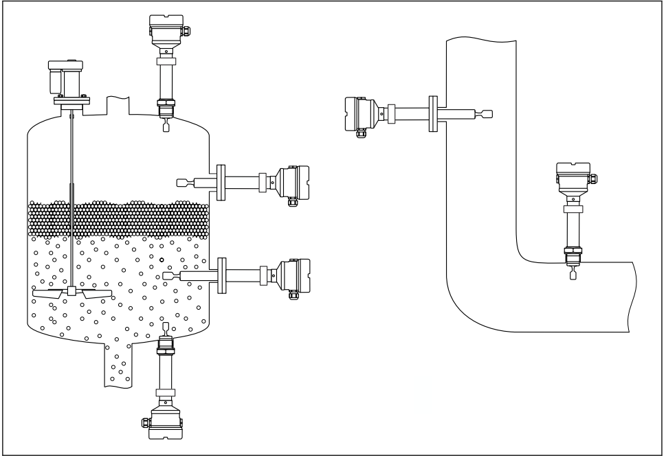
☐ 1 용기, 탱크 또는 배관에 설치 예
