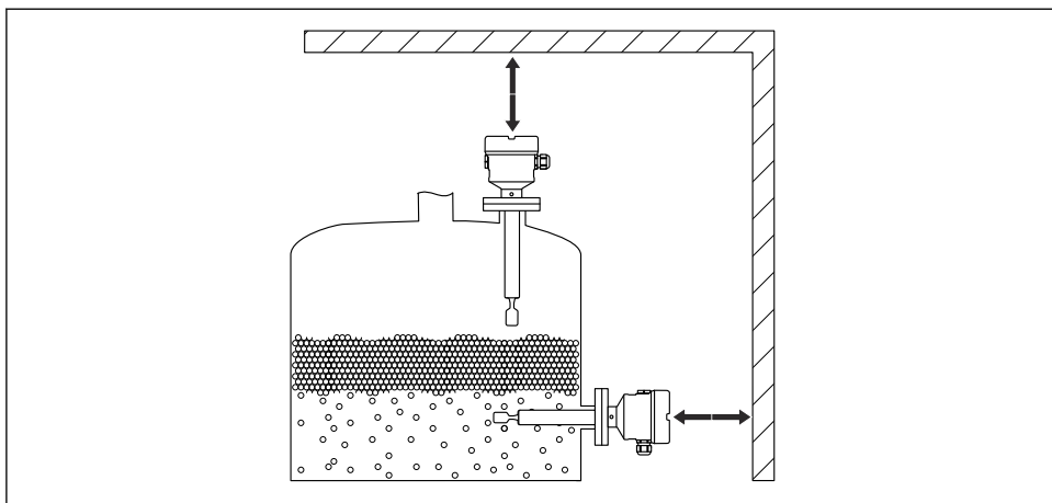
6 Zachowanie odpowiedniego odstępu
