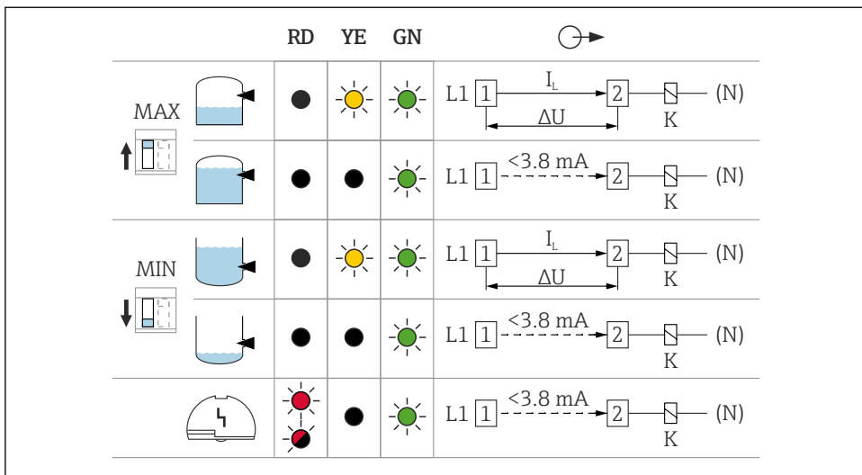
15 Reakcja wyjścia dwustanowego i sygnalizacja (wkładka elektroniki FEL61)
