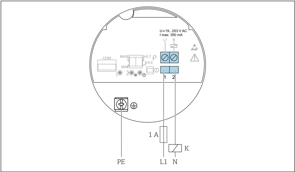
14 Wersja dwuprzewodowa AC (wkładka elektroniki FEL61)
