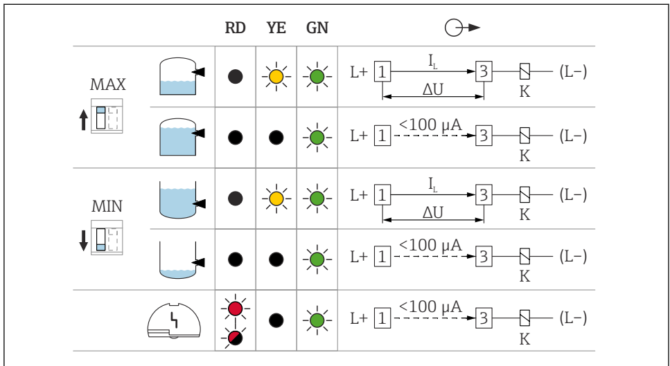
18 Reakcja wyjścia dwustanowego i sygnalizacja, wkładka elektroniki FEL62
