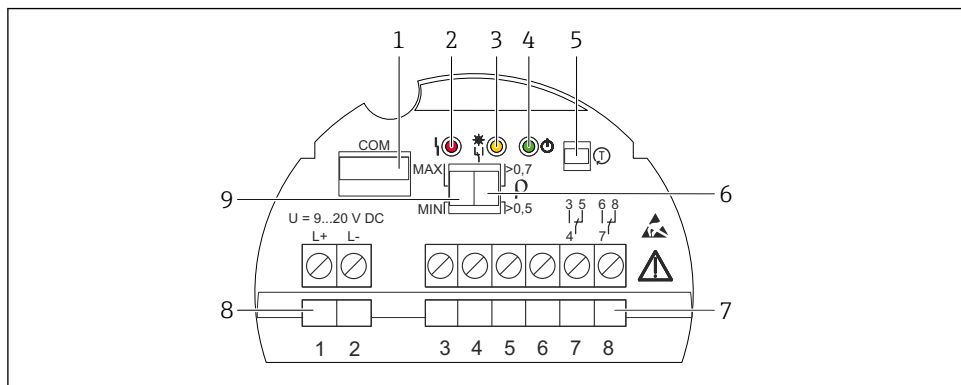
28 Przykład: wkładka elektroniczna FEL64DC
