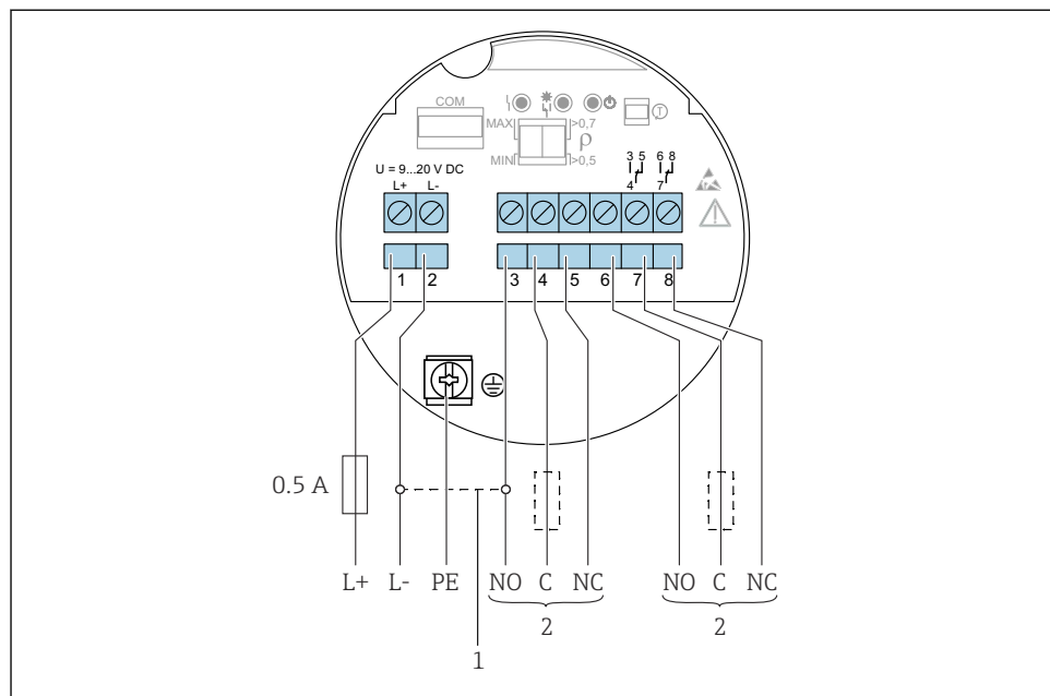
21 Wersja DC z wyjściem przekaźnikowym, wkładka elektroniki FEL64 DC
