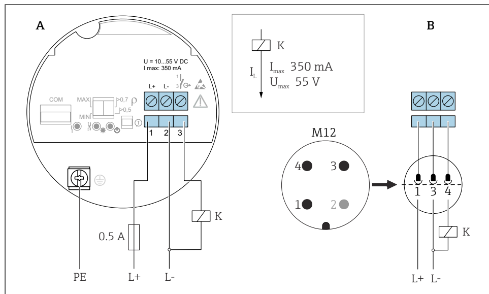
17 Wersja 3-przewodowa DC z wyjściem PNP (wkładka elektroniki FEL62)
